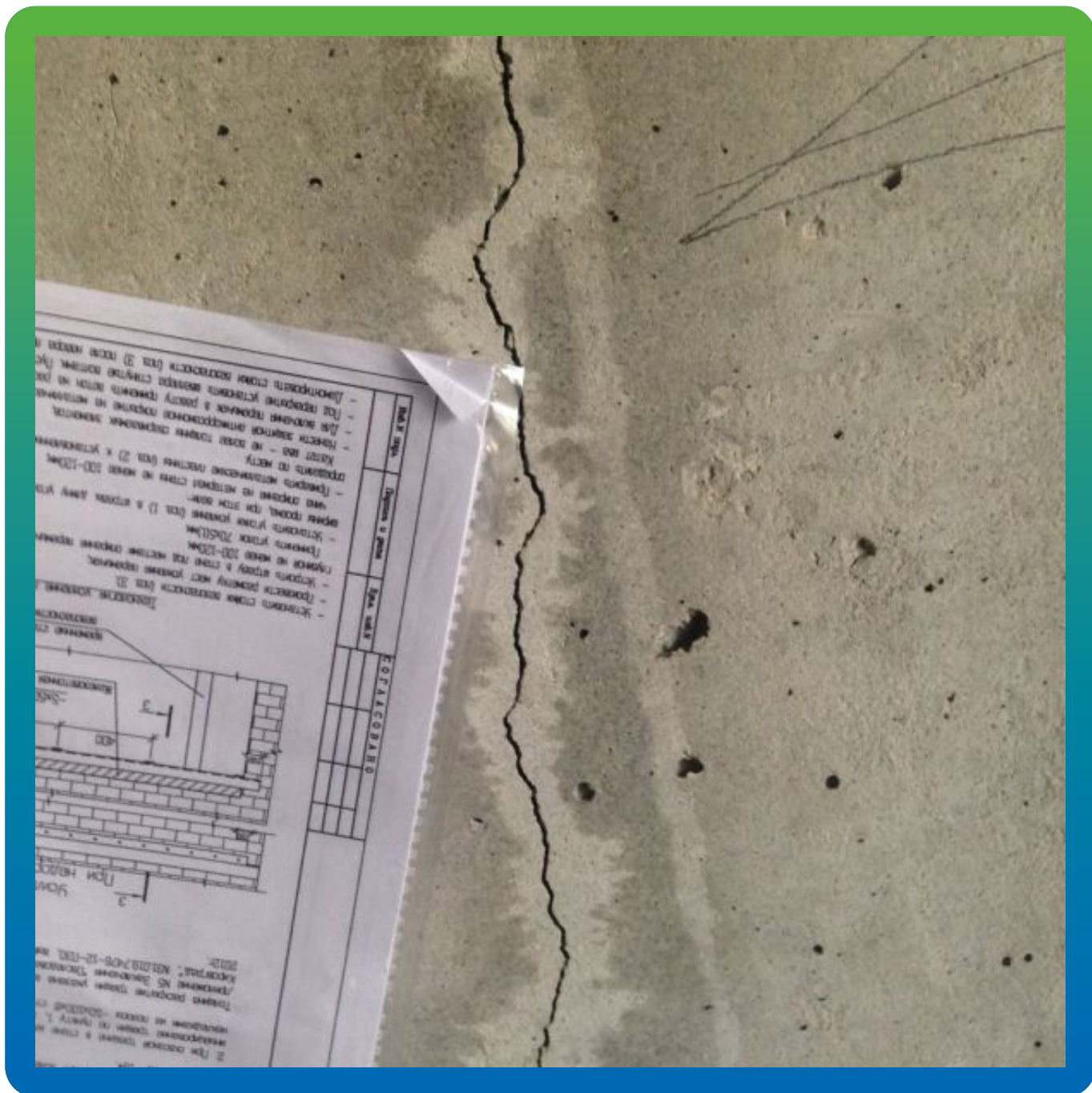
Вид дефектов.
