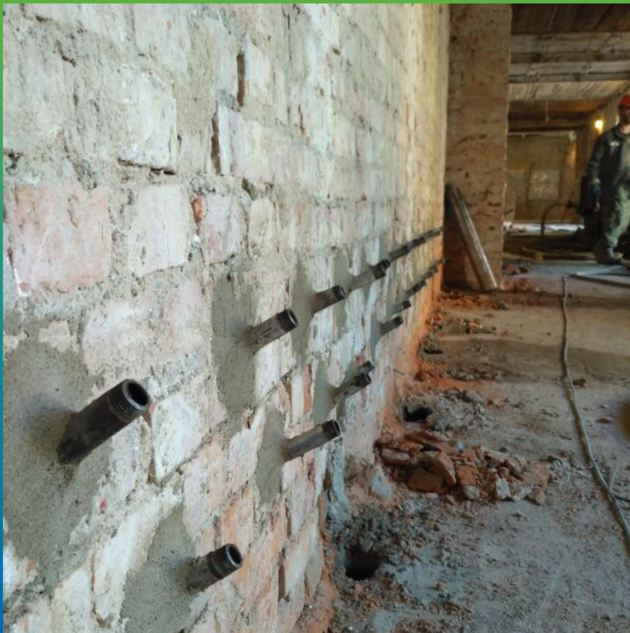
Монтаж инъекторов
