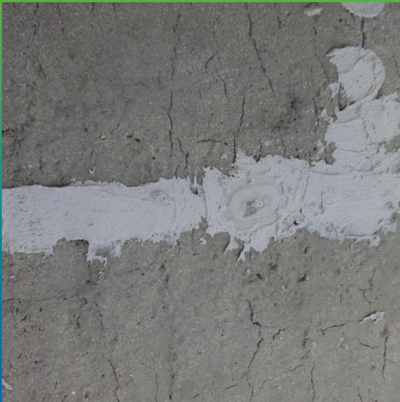
Установка пакеров БМ 0187
