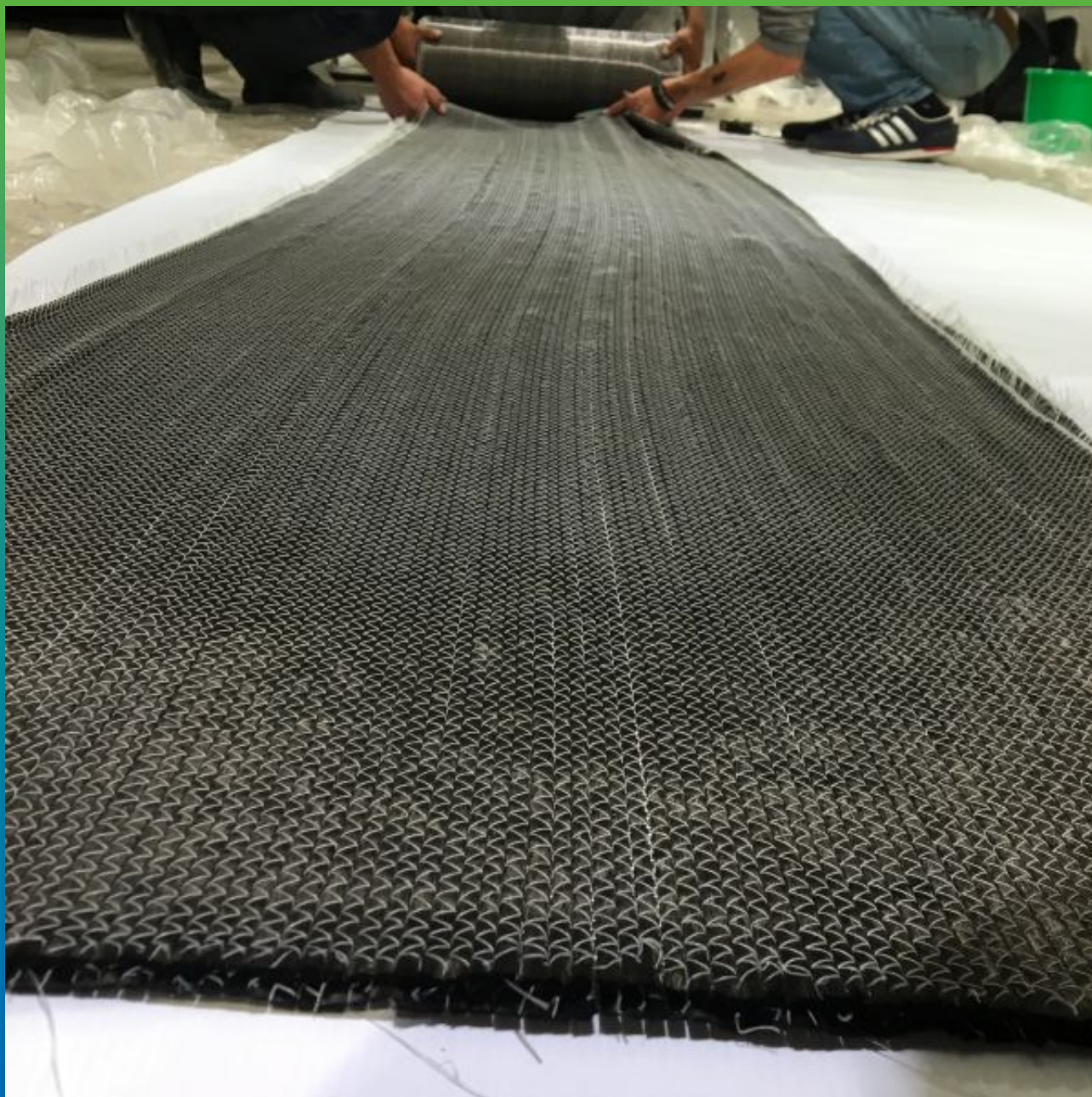
Раскрой материала Армошел KB 500
