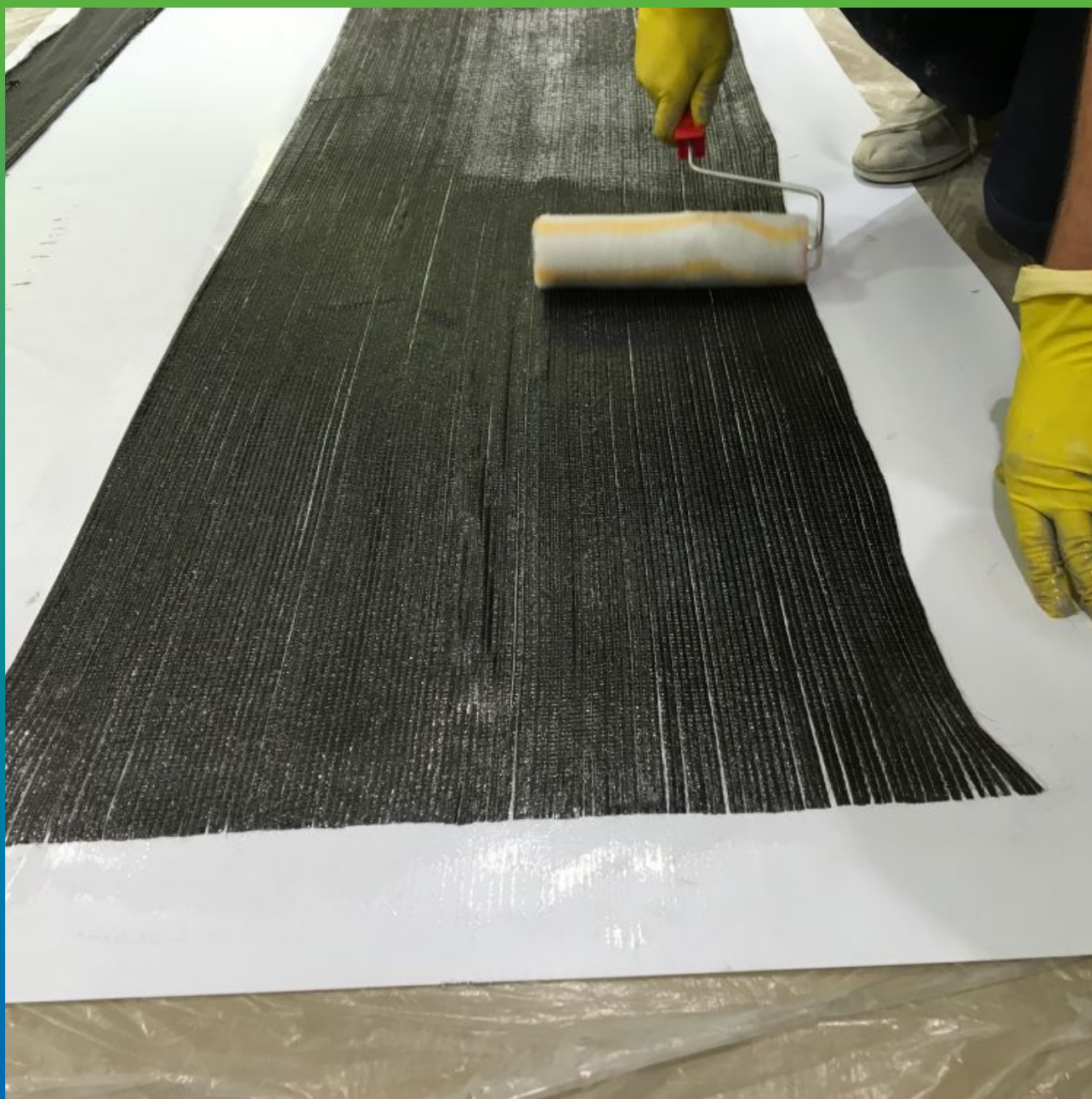
Пропитка углеволоконного холста Армошел 500
