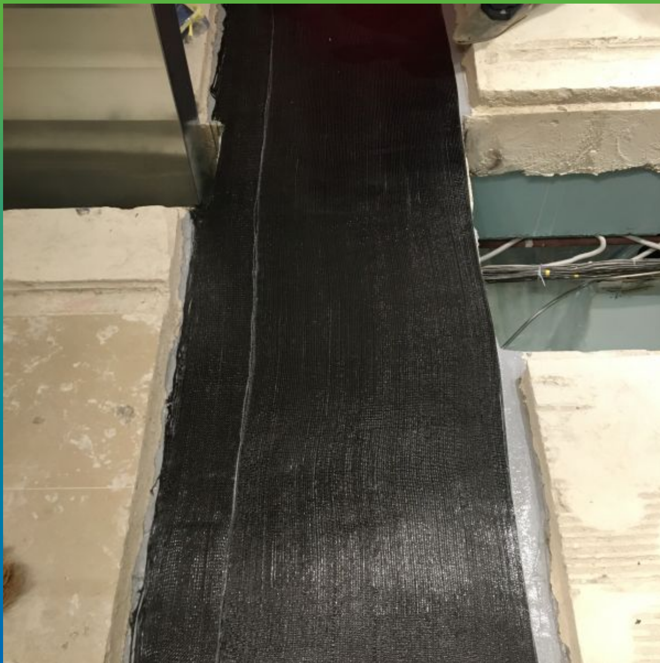
Монтаж углеволоконного холста Армошел 500
