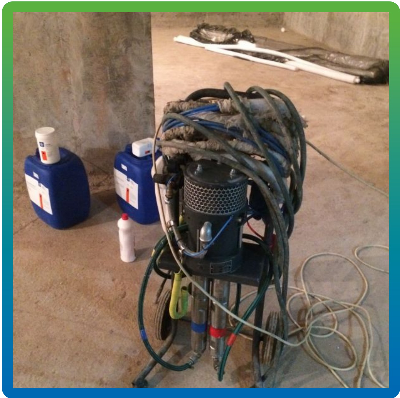
Инъекционный пневматический насос БМ 1425 на объекте
