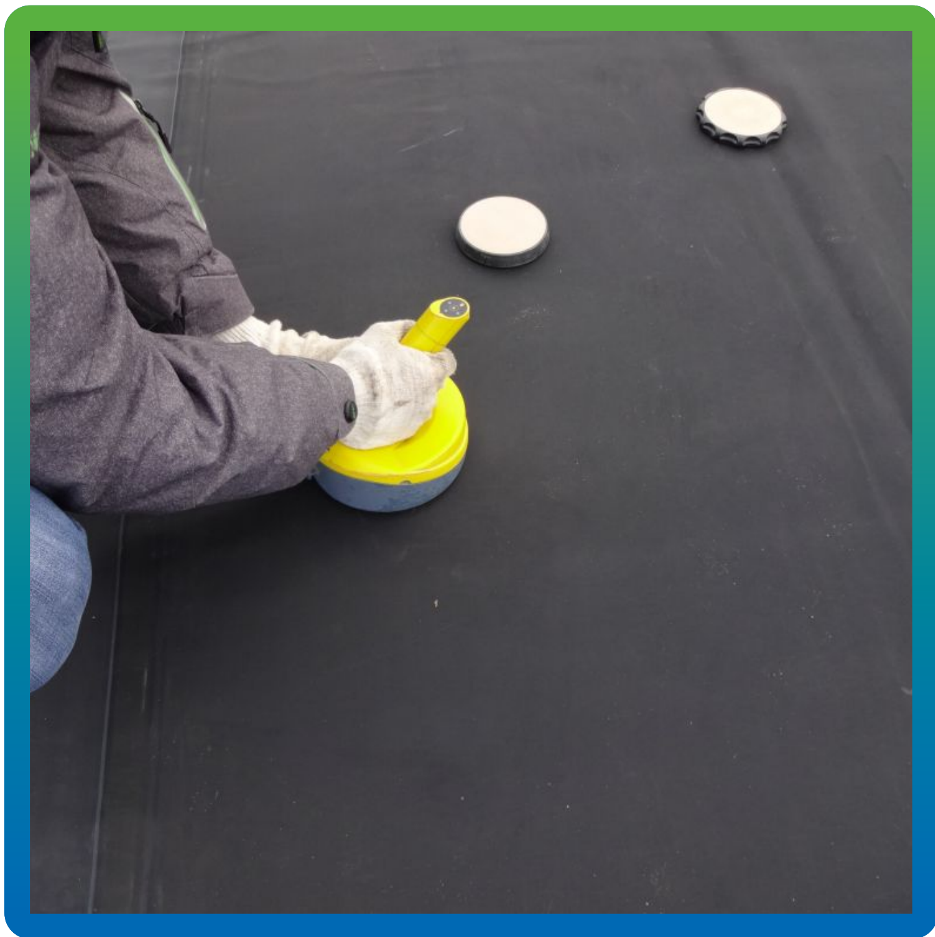
Приваривание шайб к мембране по технологии "Центрикс"
