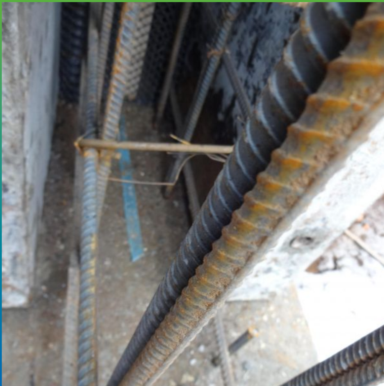
Уложенный профиль Манодил Свелл, перед заливкой бетона с добавкой Реолен Адимкс
