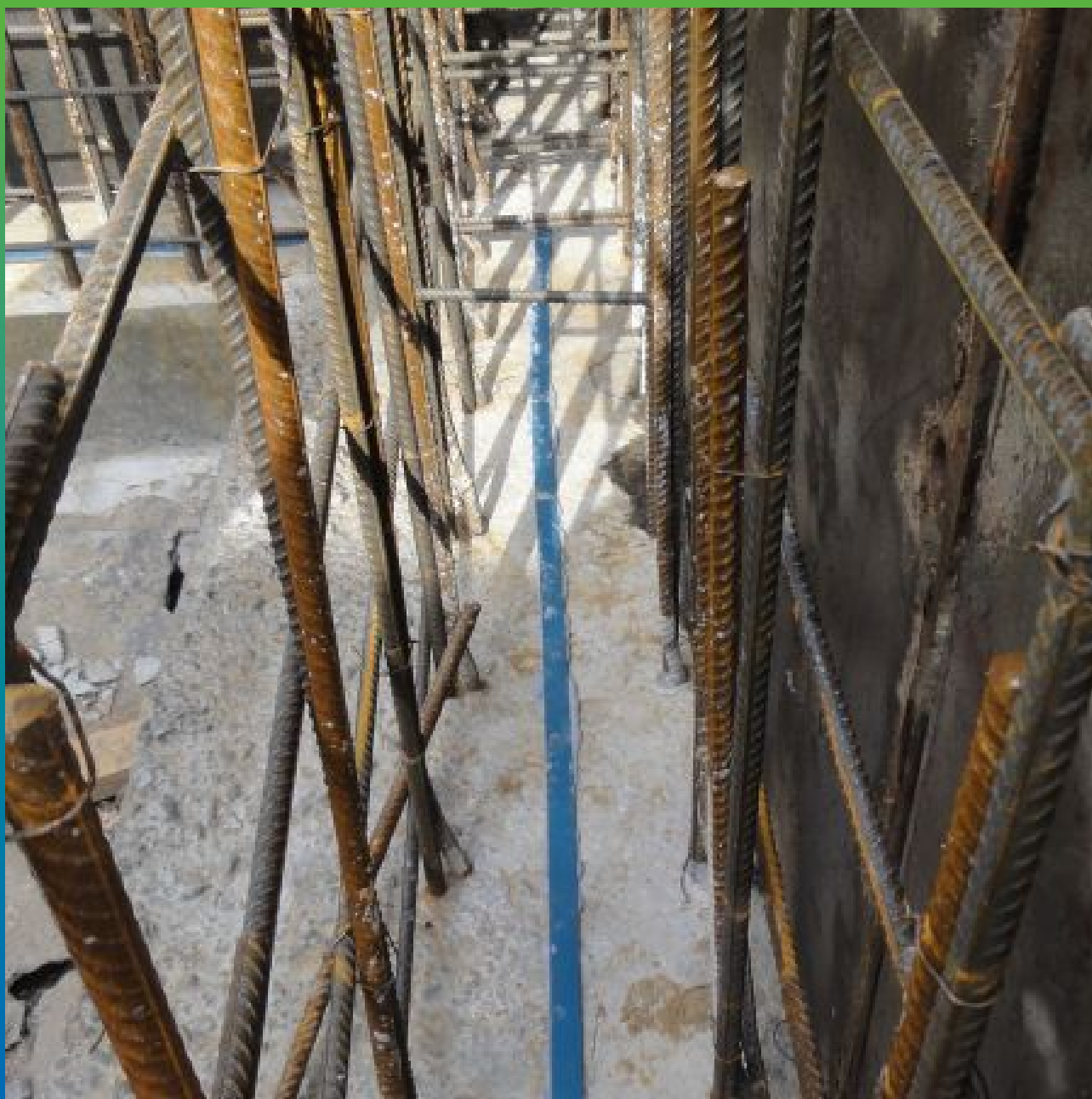
Укладка гидрофильного профиля Манодил Свелл на расширяющийся герметик Манодил Свеллмастер
