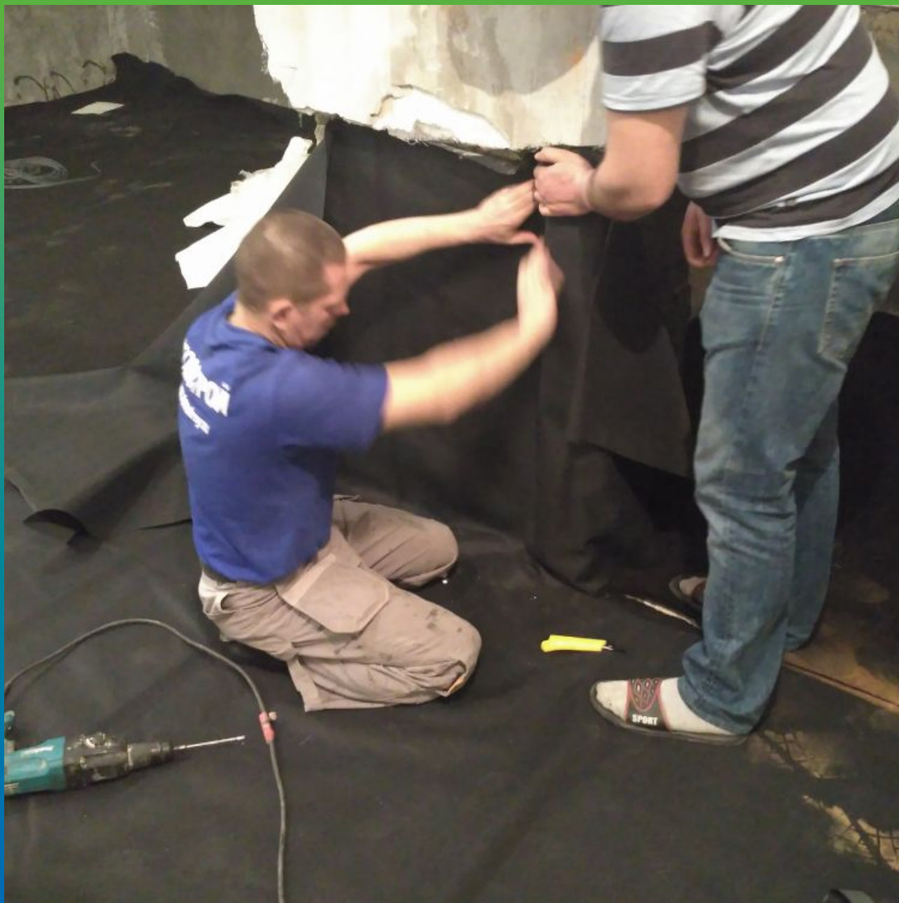
Приклеивание мембраны к вертикальным поверхностям с клеящим составом Адгезив П-400
