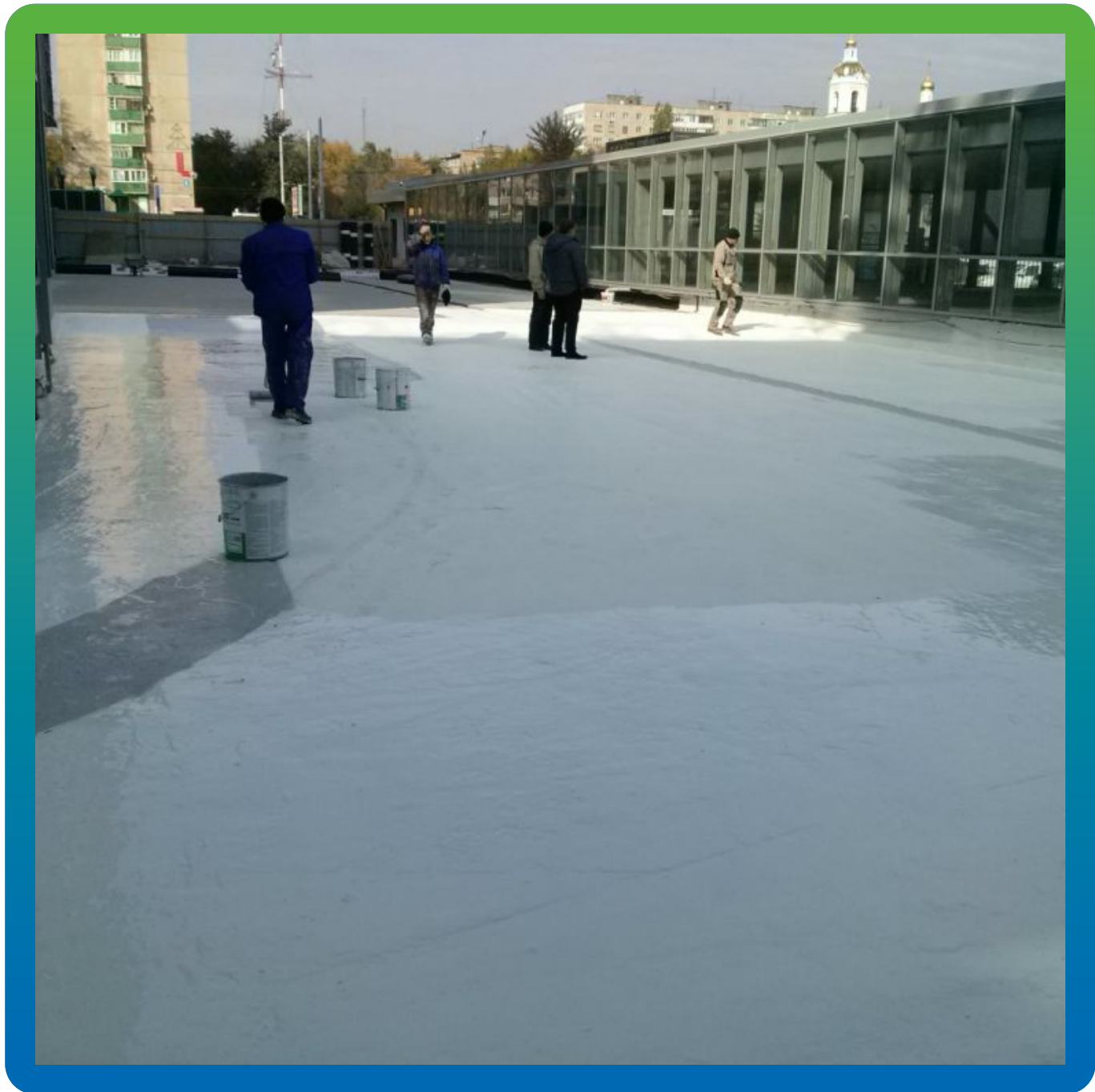
Нанесение второго слоя гидроизоляции Максэластик Пур
