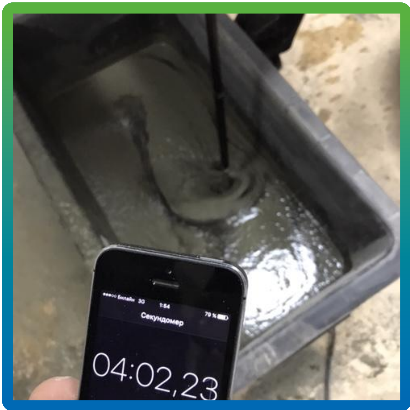
Подготовка состава к заполнению опалубки
