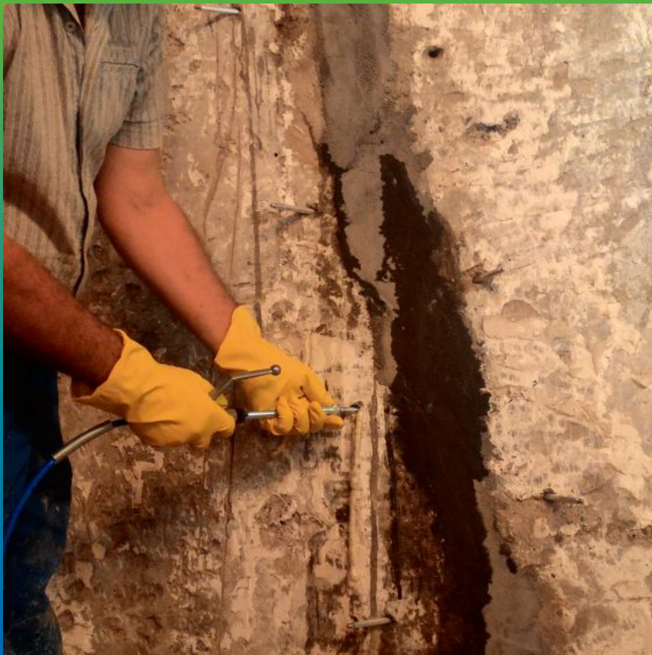
Процесс инъектирования состава Манопур 15 с последующим инъектированием Манопур 143
