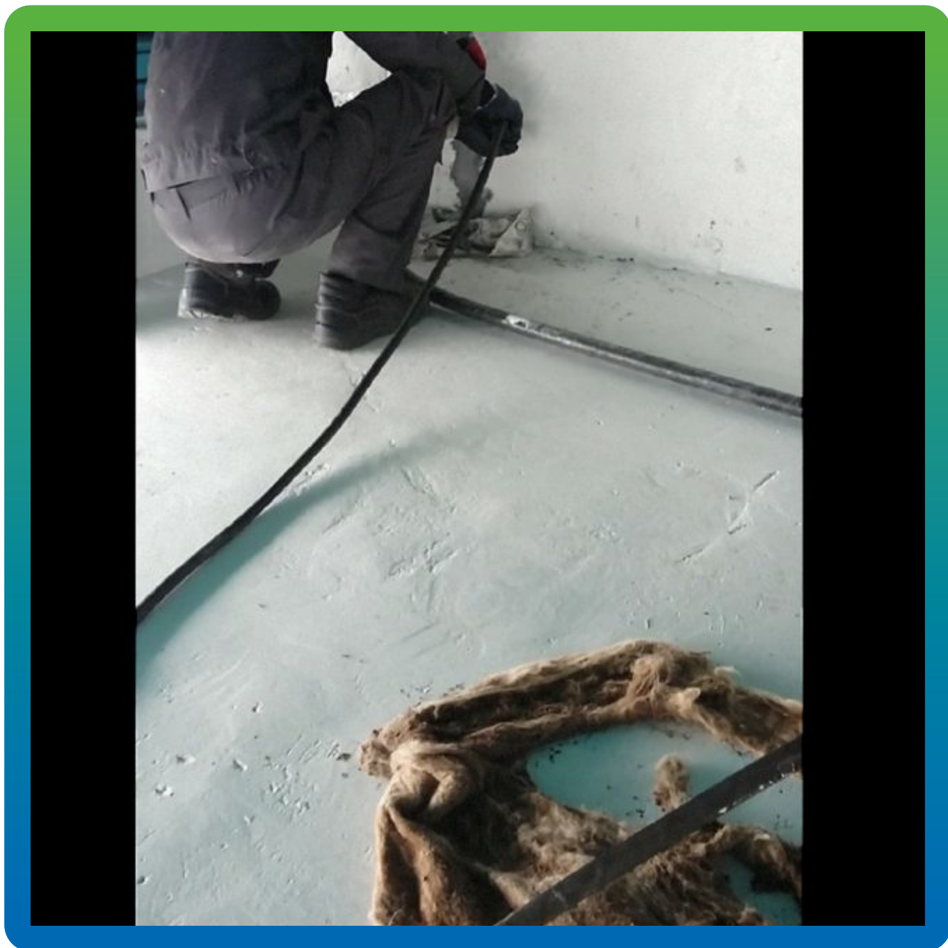
Инъектирование в трещины и швы эпоксидного состава Манопокс 352
