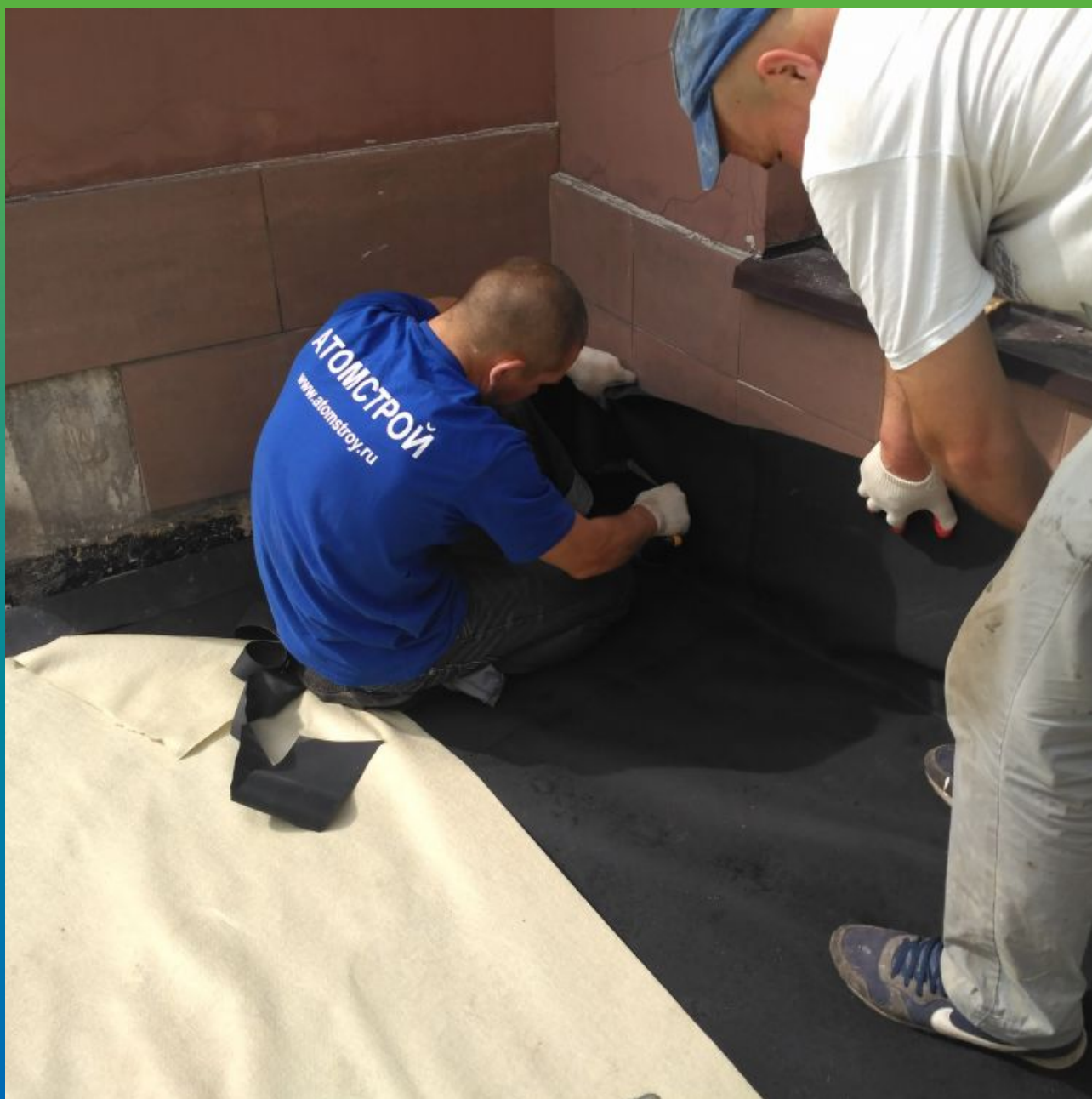
Устройство примыканий
