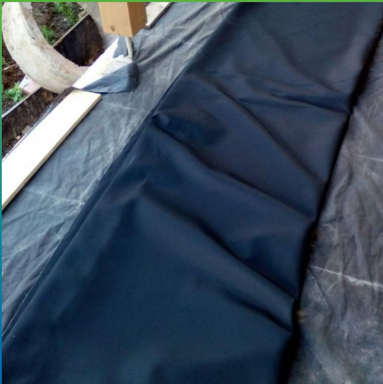
Укладка ЭПДМ мембраны Преласты СТ
