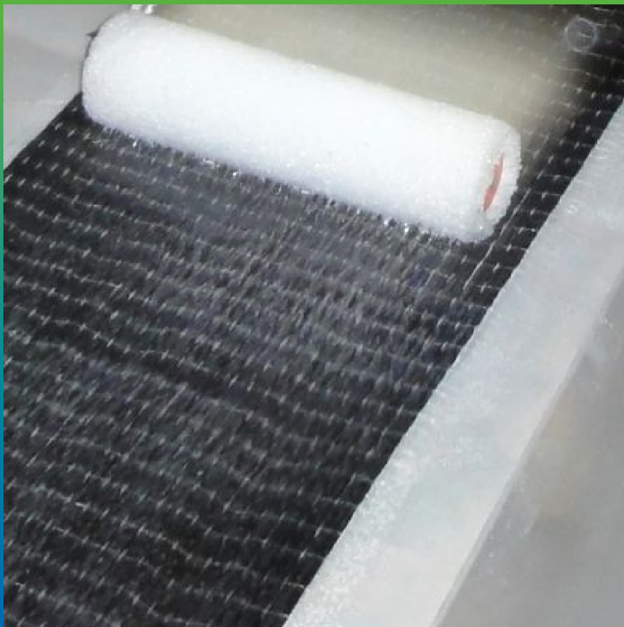
Пропитка ткани клеем Манопокс 372.
