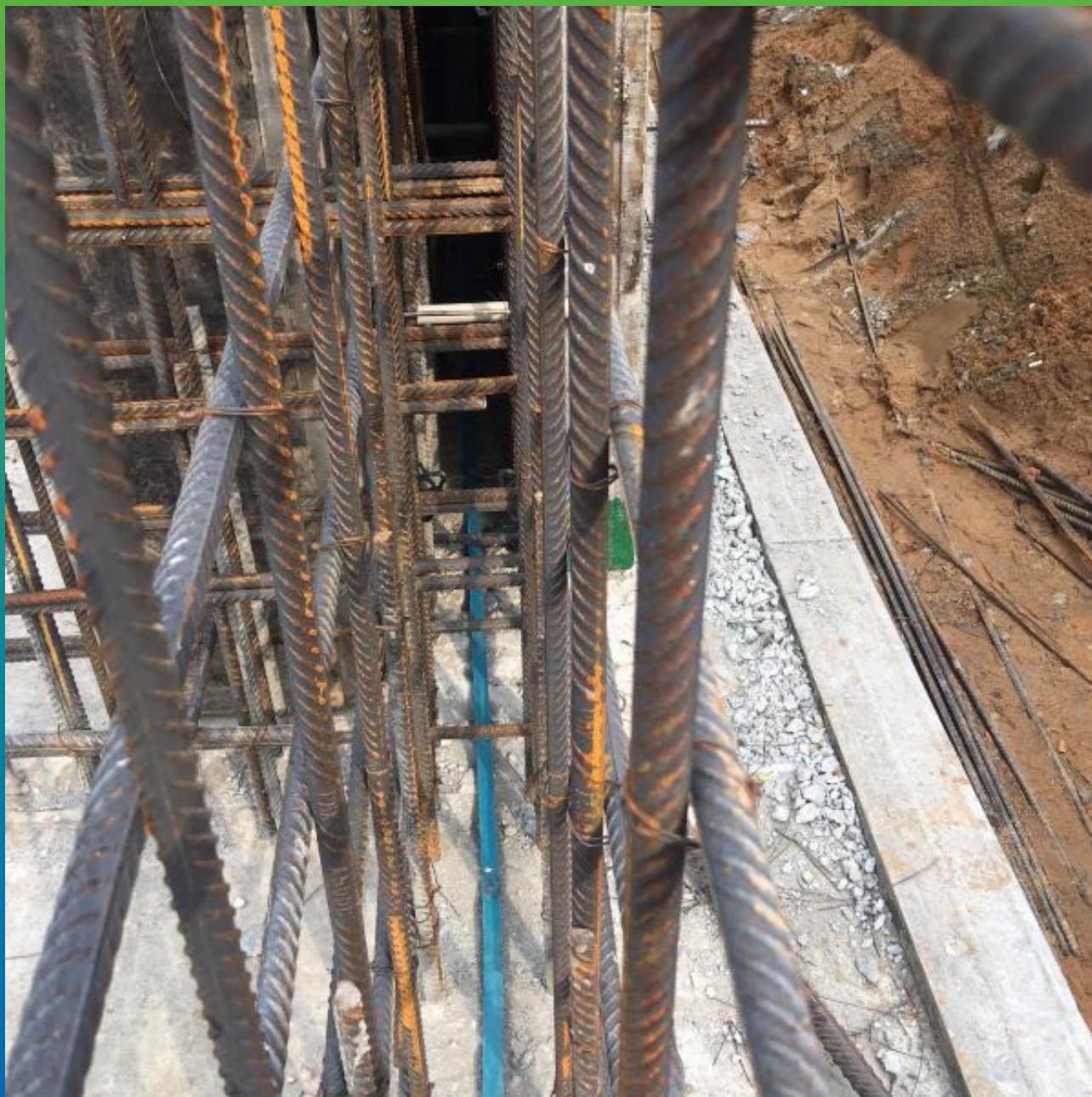
Укладка профиля Манодил Свелл ХК 2507
