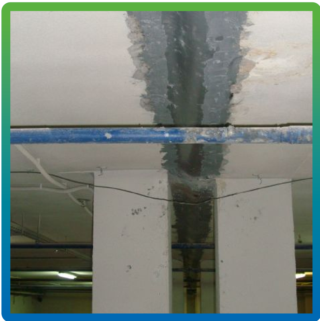
Вид выполненного деформационного шва
