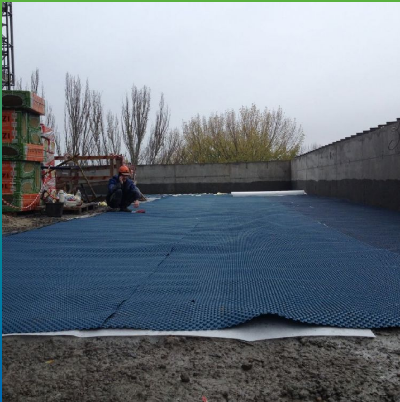
Раскладка дренажного полотна Максдрейн 8 по геотекстилю
