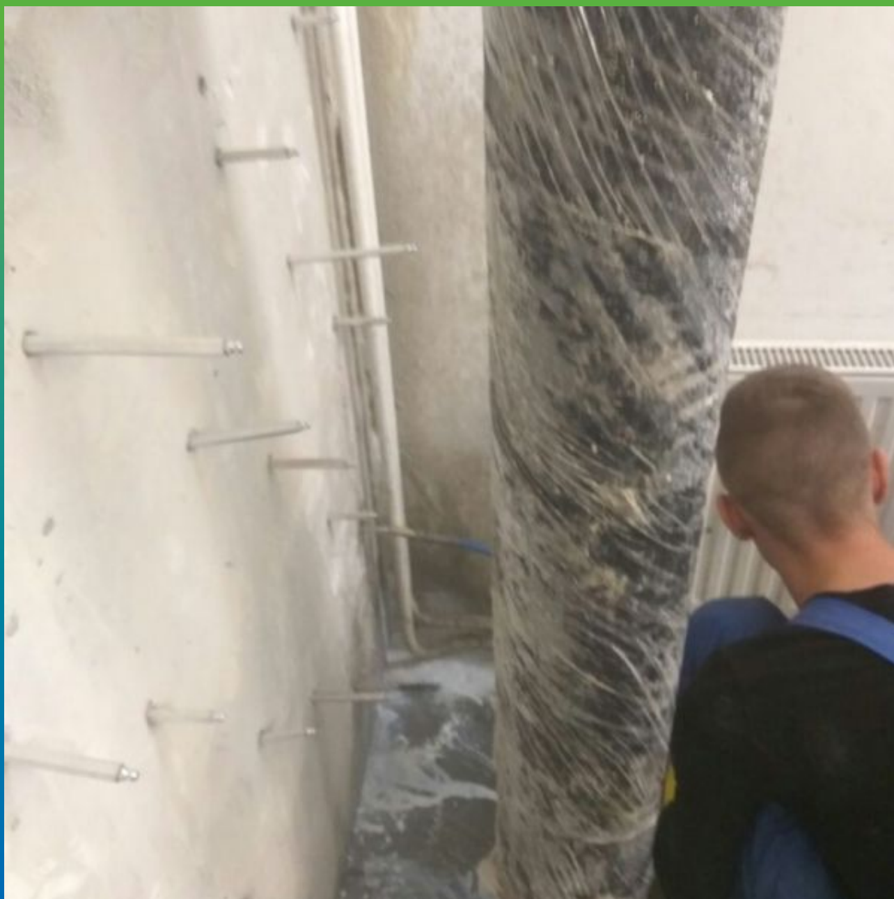
Установленные пакеры
