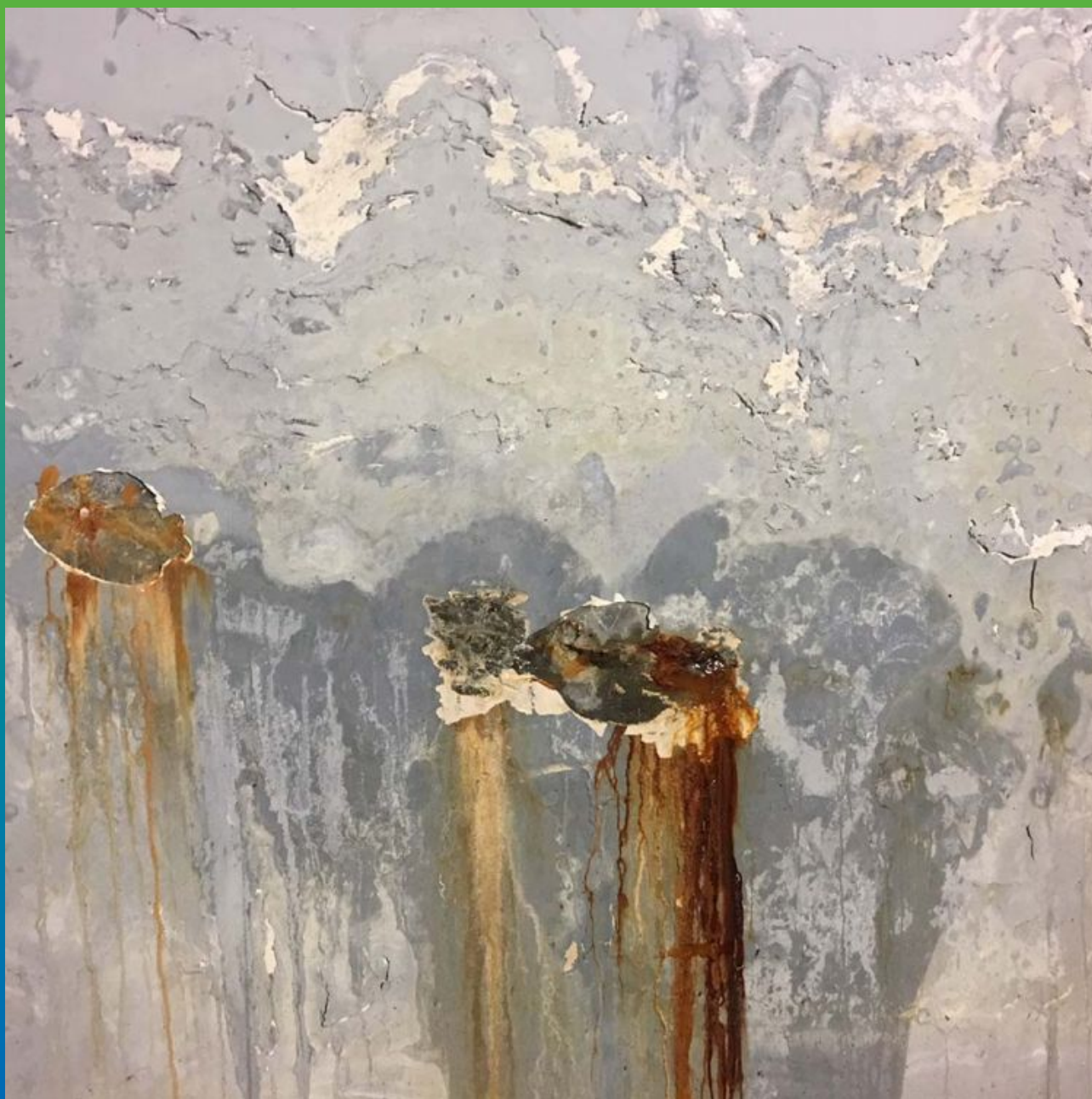
Виды дефектов на паркинге
