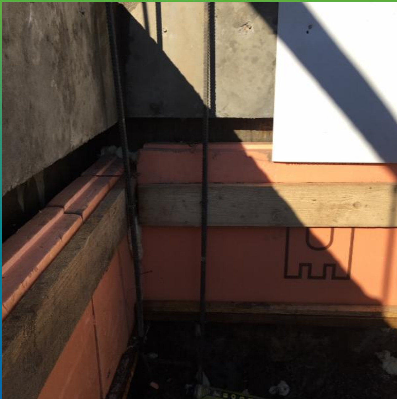
Вид шва между стеной в грунте и утеплителем
