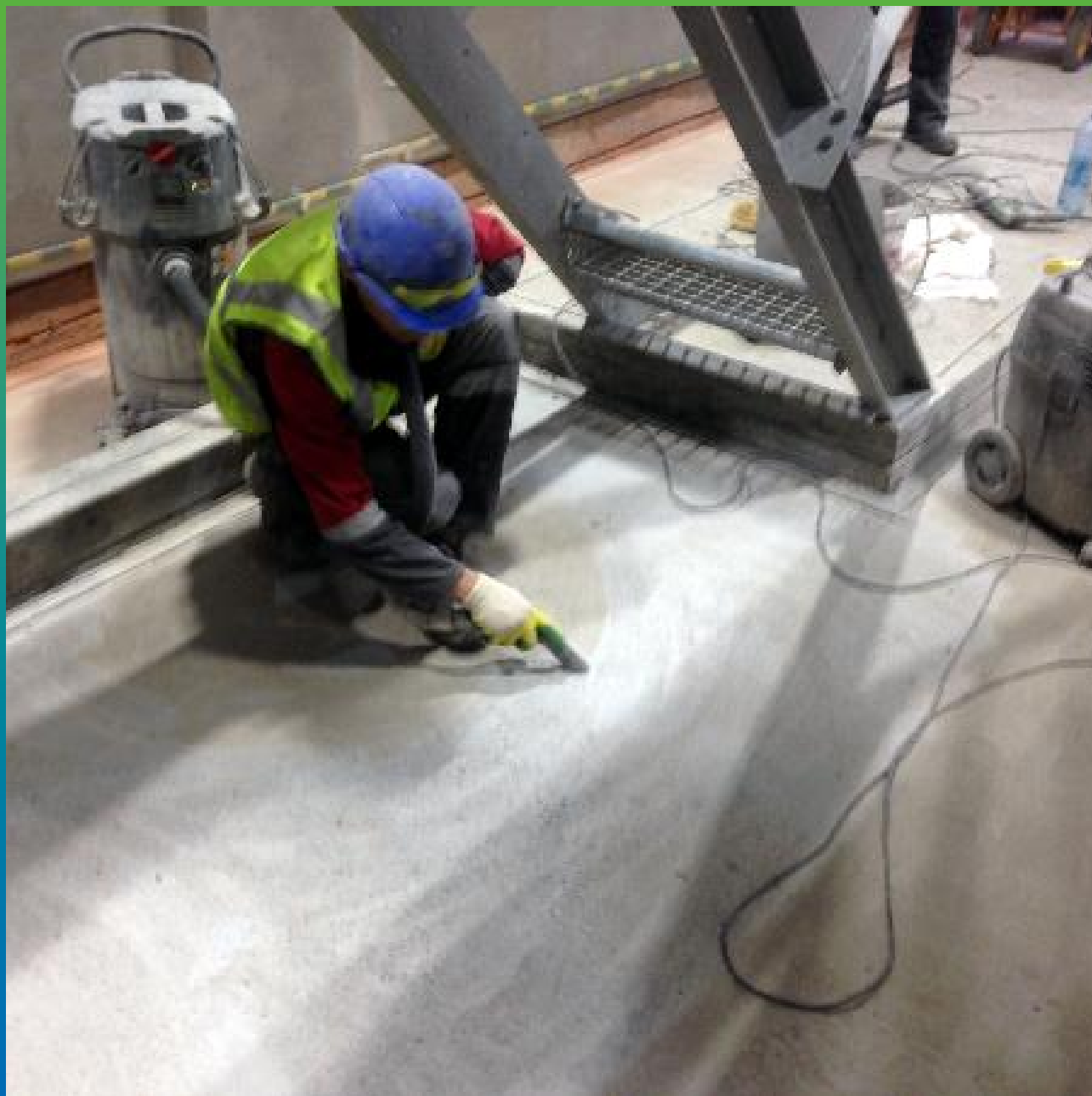
Подготовительные работы. Обеспыливание промышленными пылесосами.
