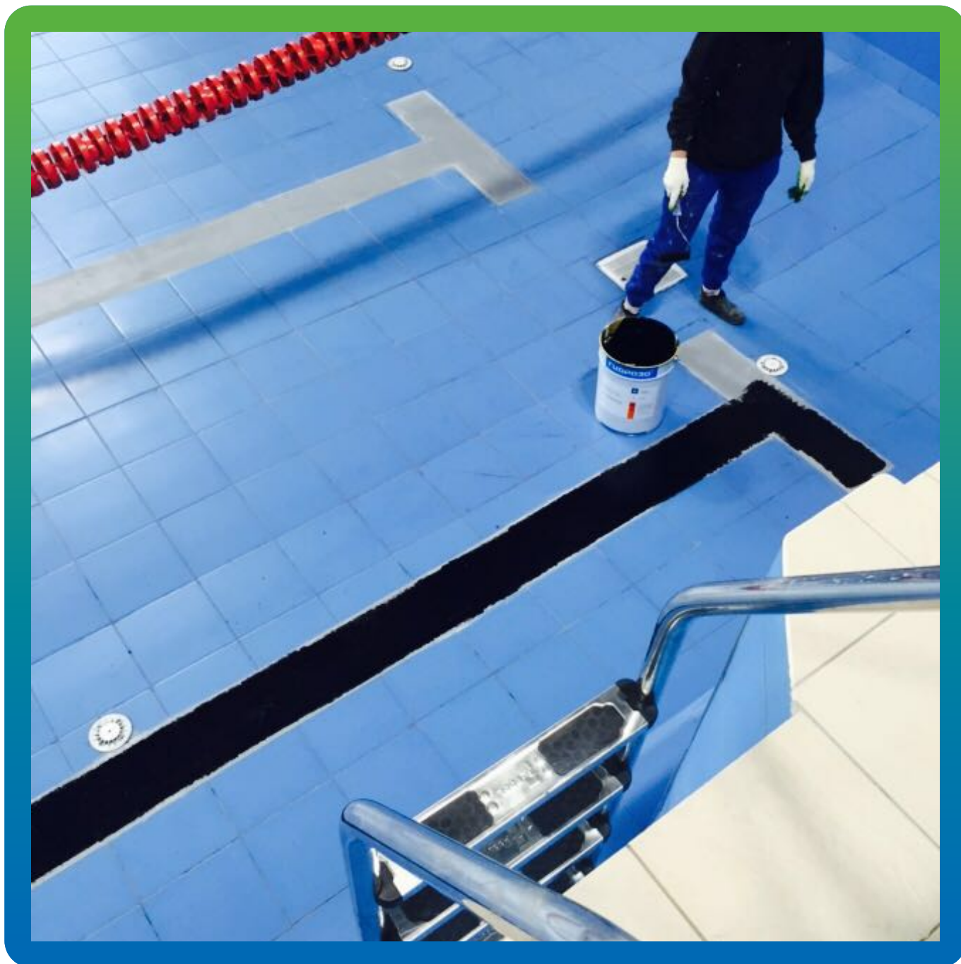
Нанесение материала Денстоп ЭП 201 на подготовленные участки выполненные материалом Манопокс 331
