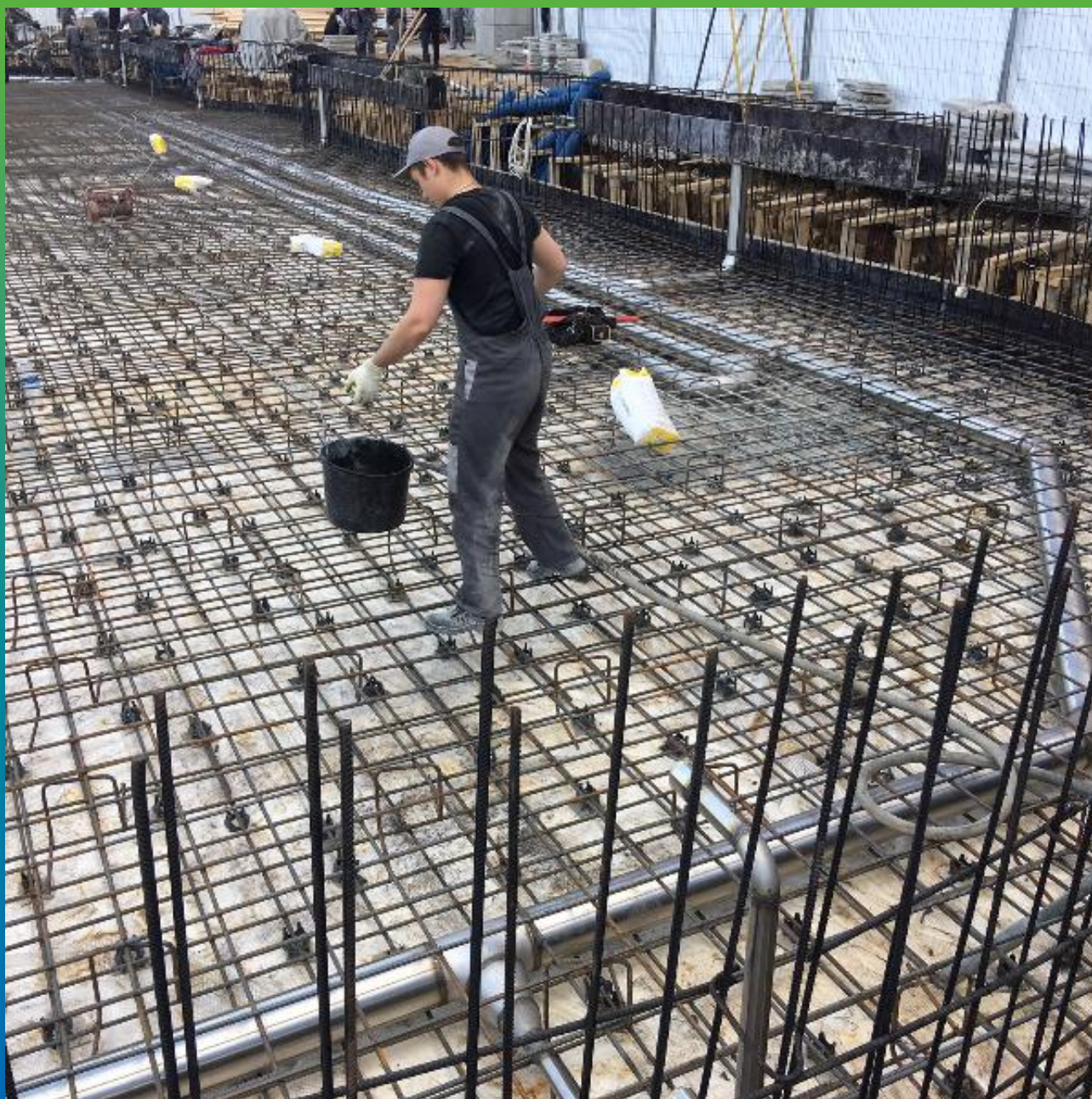
Просыпка материала Стармекс Сил перед отливкой плиты
