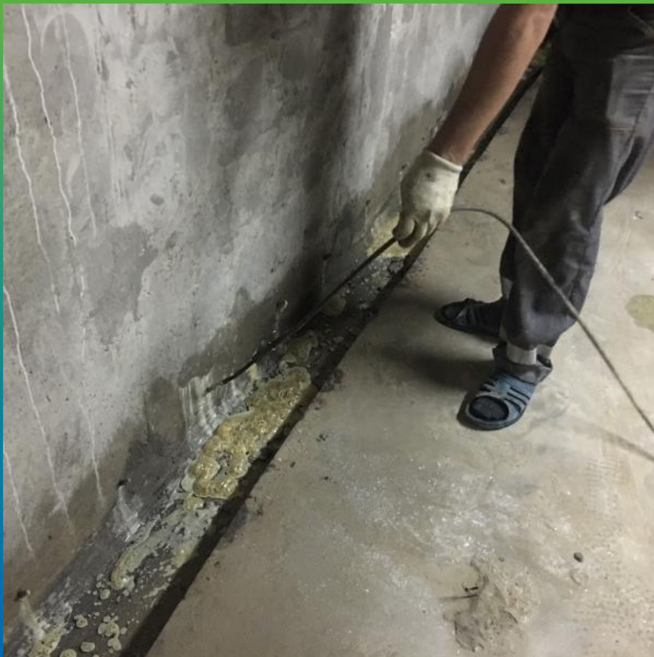
Инъектирование в шов полиуретановой смолы Манопур 143
