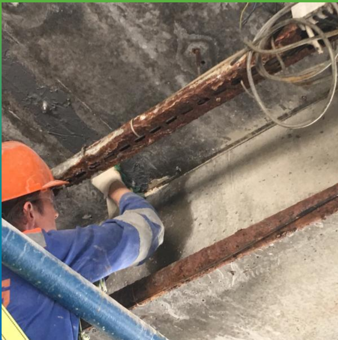
Установка пакеров БМ 0189 по межплиточным швам на Манопокс 331
