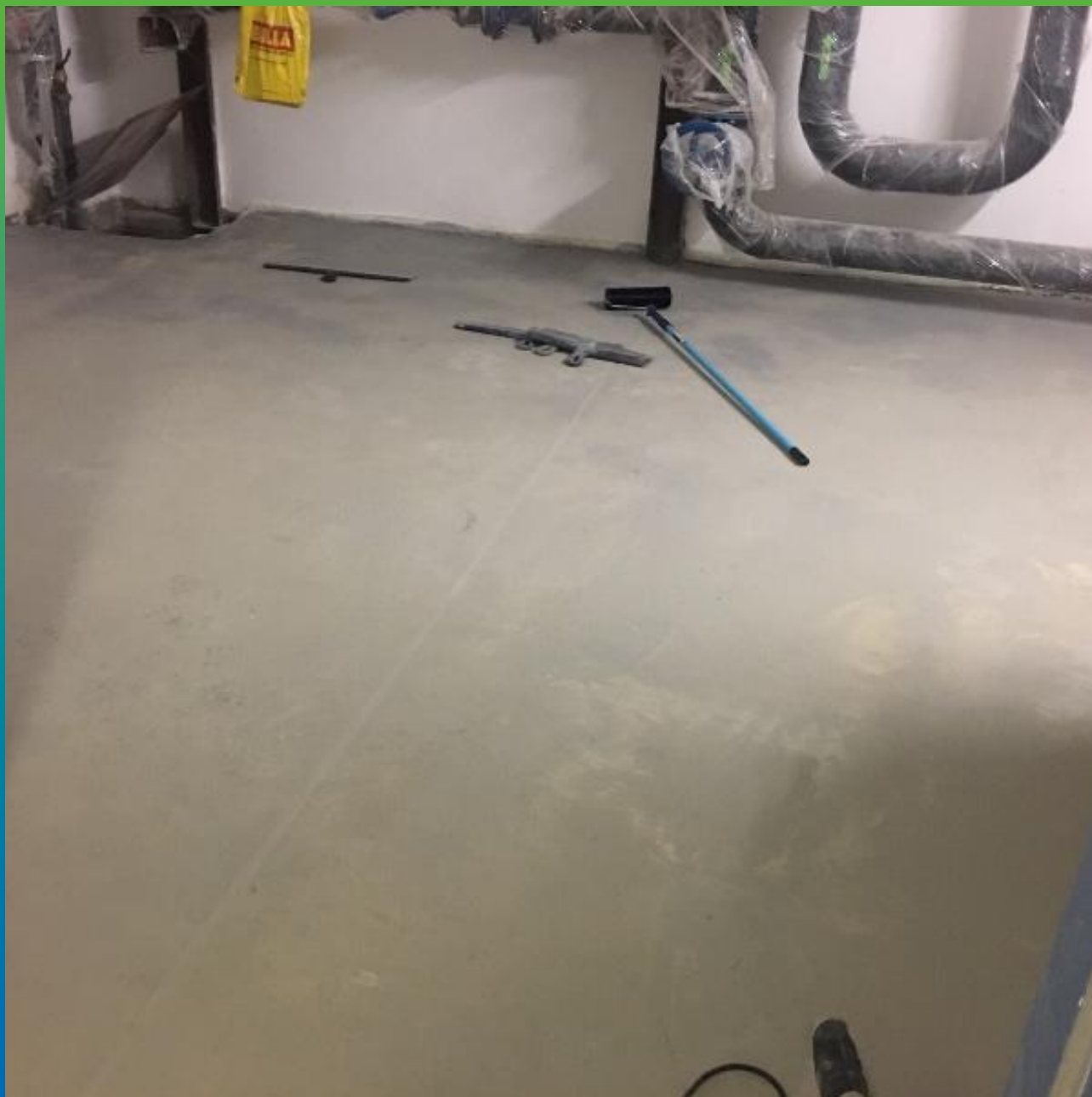
Вид подготовленного основания, грунтовка ДенсТоп ЭП 105 с песком ДенсТоп Филлер
