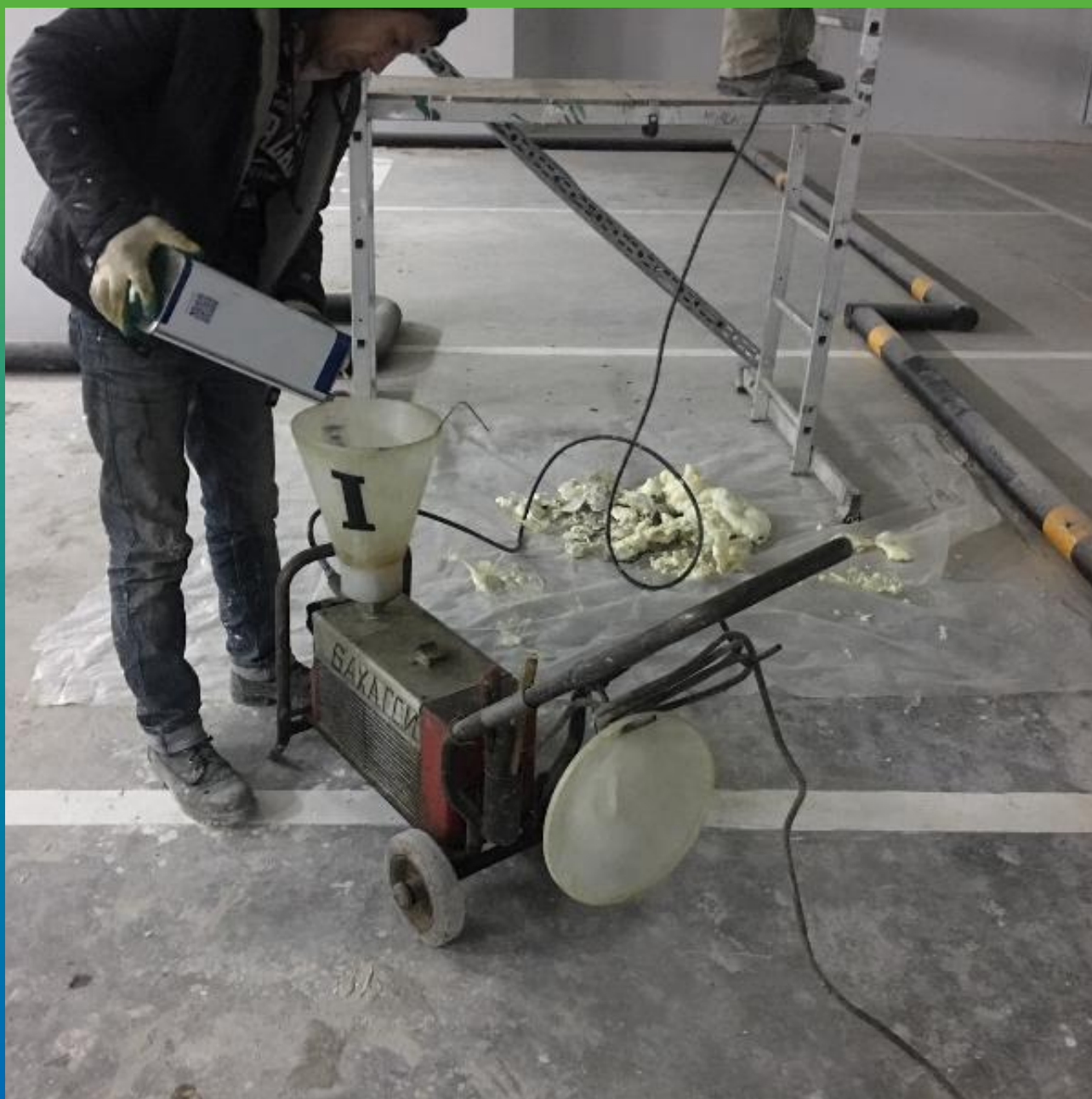
Подача материала Манопур 143 в инъекционный насос
