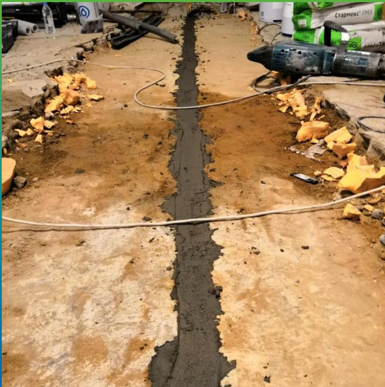
Зачеканка шва ремонтным составом Стармекс РМЗ
