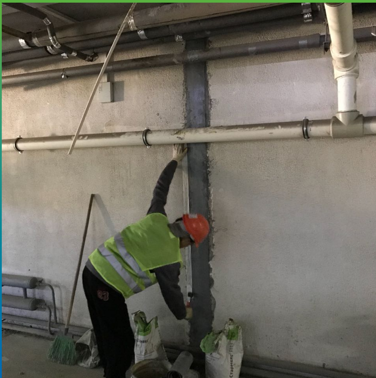
Монтаж гидроизоляционной ленты Манодил Про на эпоксидный клей Манопокс 331
