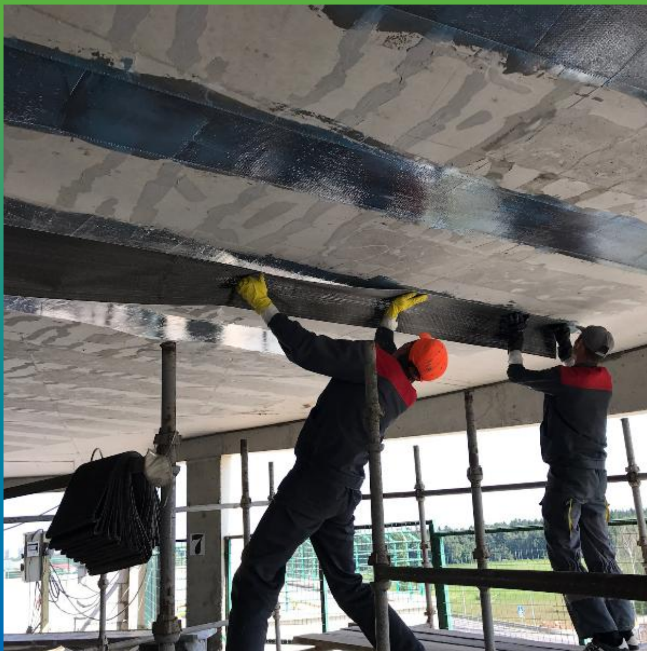
Приклеивание углеродного холста
