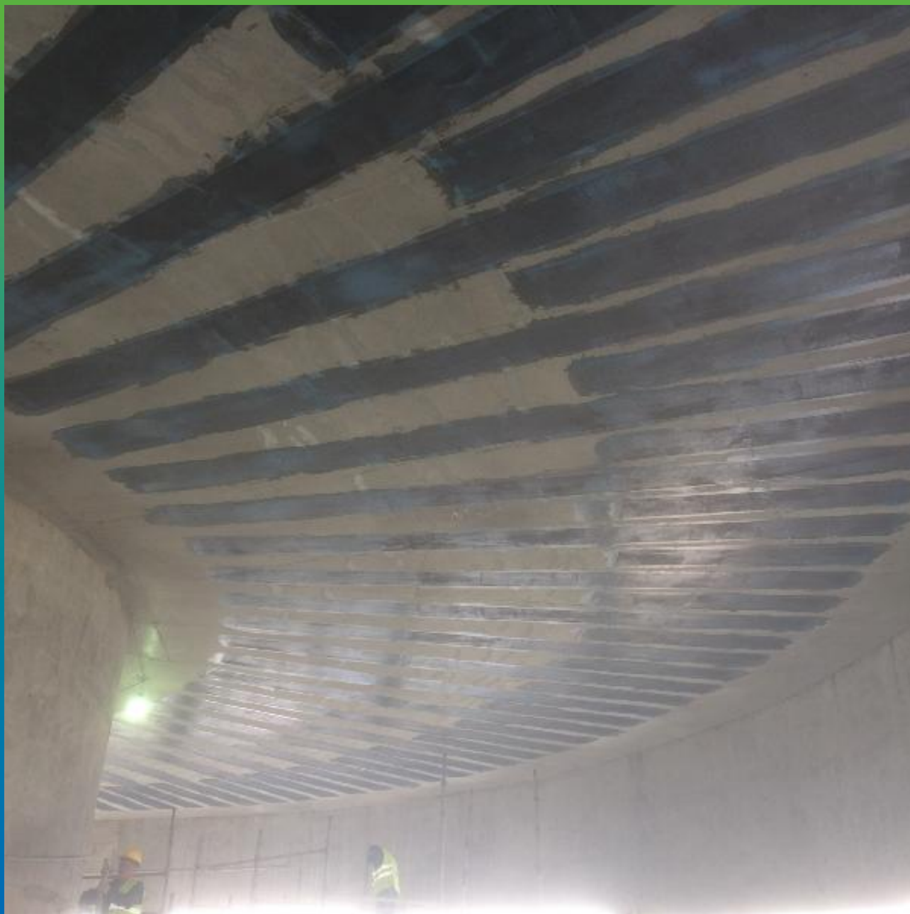
Усиленные плиты в зоне въезда
