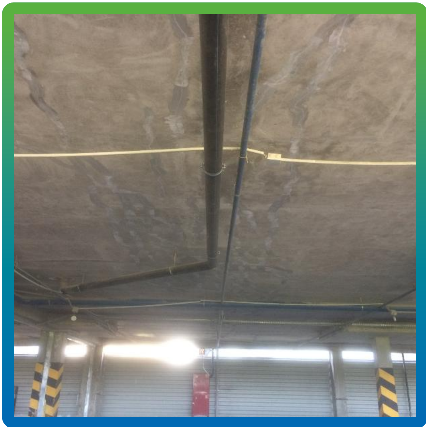
Отремонтированные трещины в плите перекрытия
