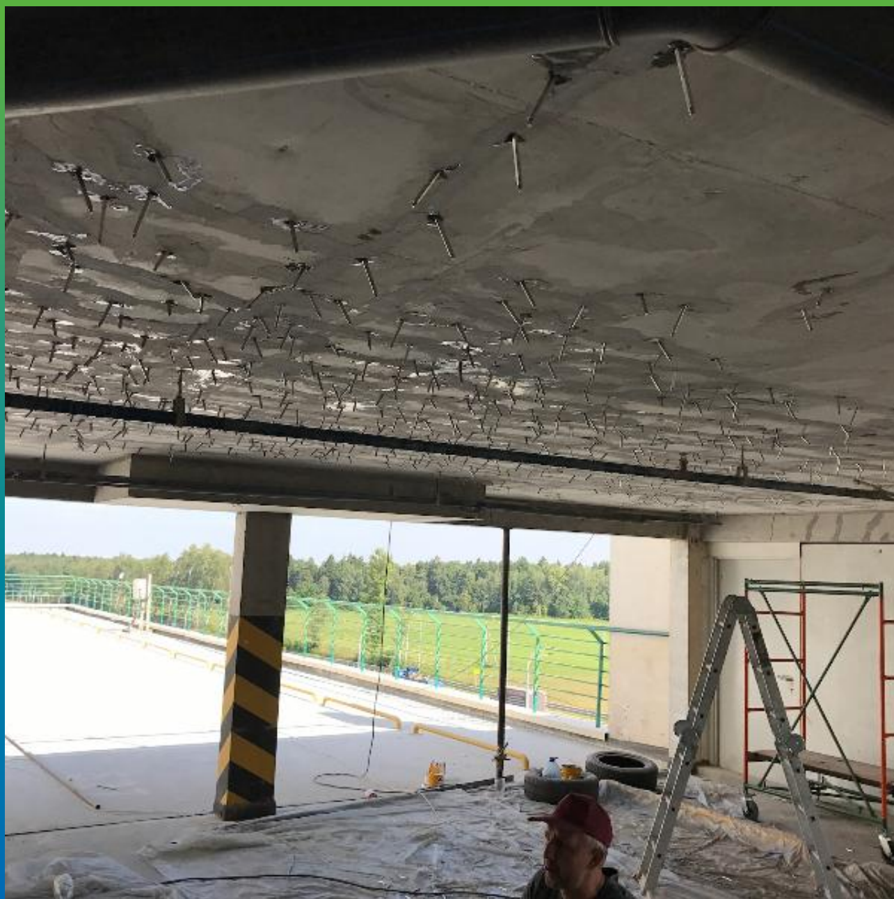
Установленные пакеры для инъектирования трещин
