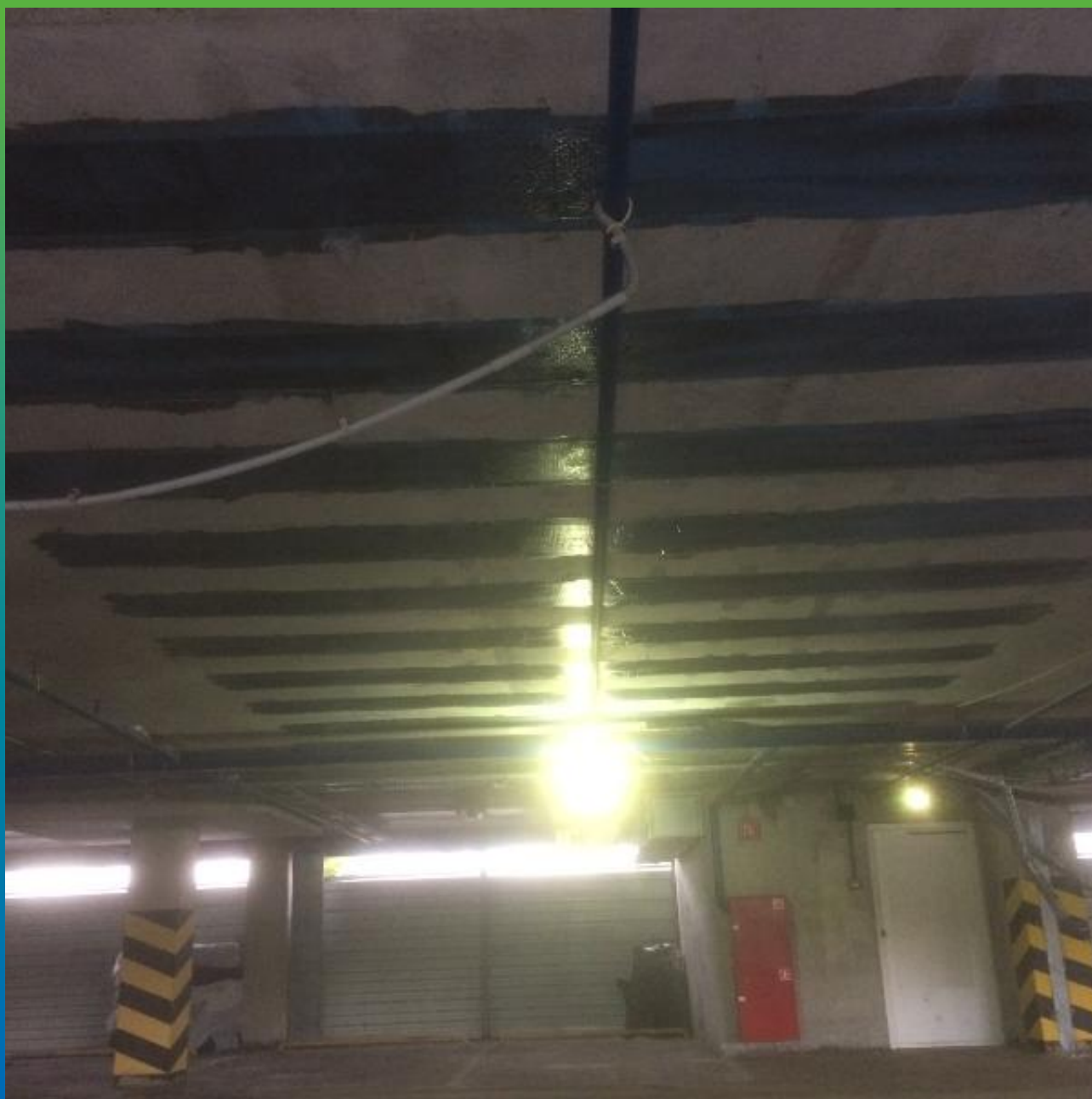
Усиленная плита перекрытия паркинга
