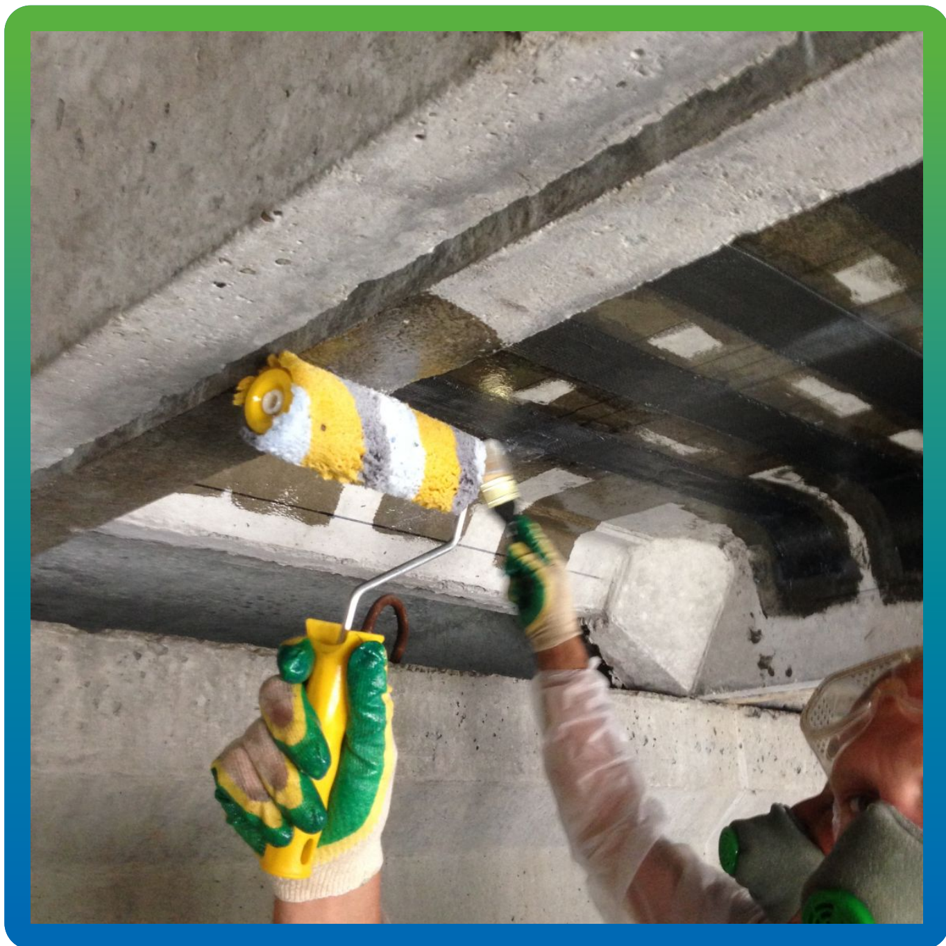
Подготовка основания. Грунтование основания составом Манопокс 372
