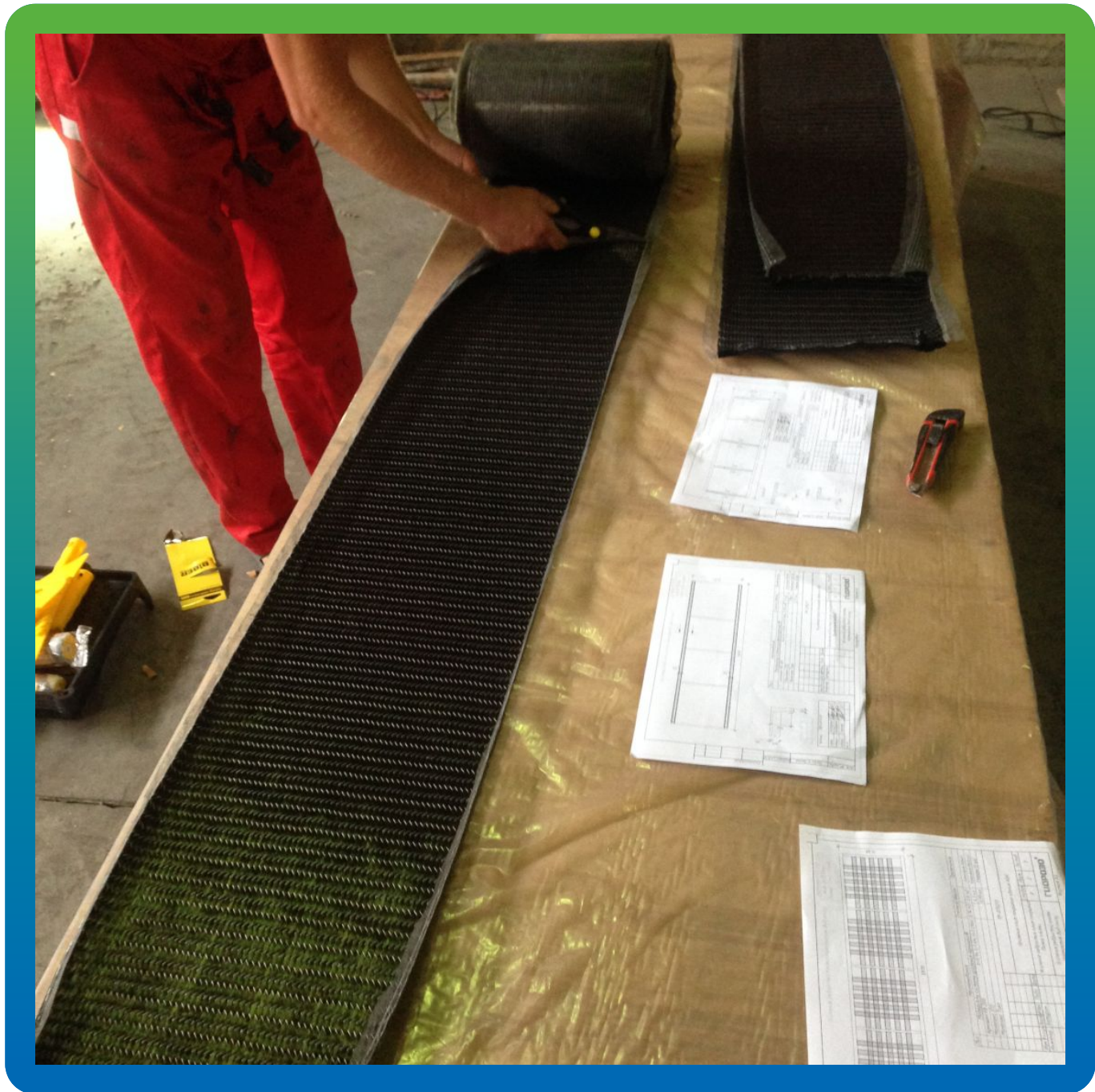
Подготовка материалов. Раскрой холста Армошел по проекту
