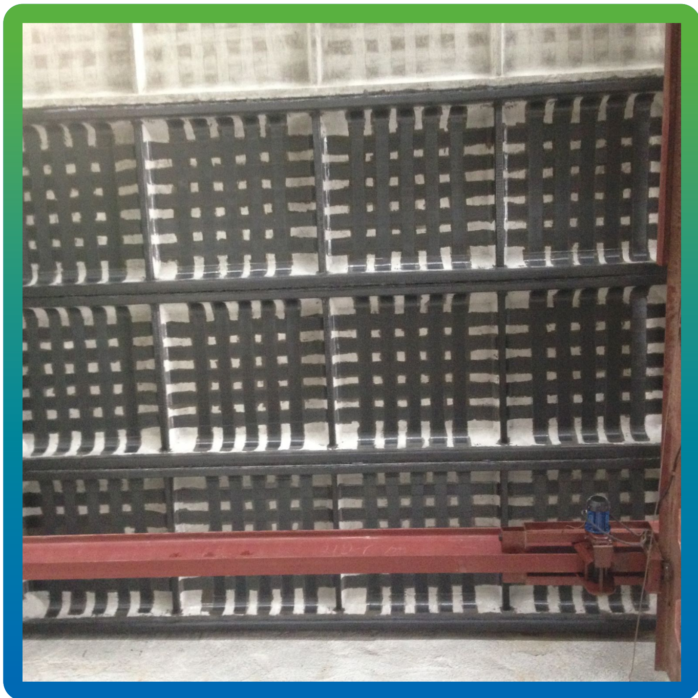
Внешний вид усиленного участка ребристых плит
