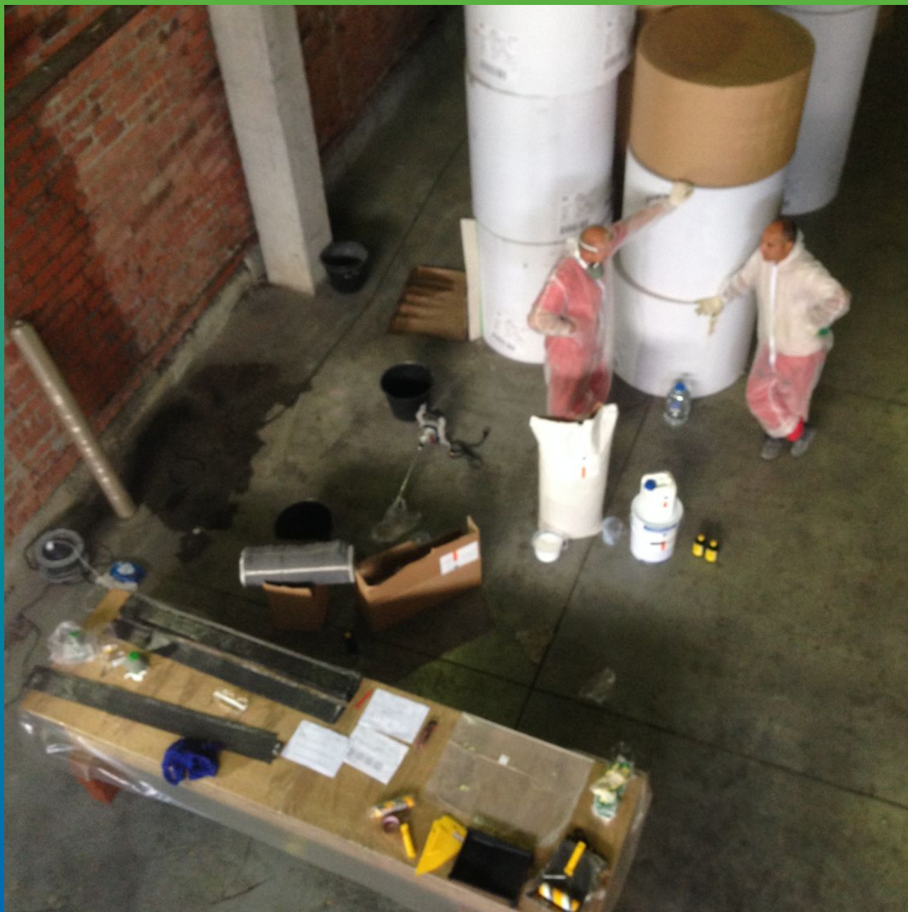
Подготовка рабочего места. Установка стола для работы с углеродными холстами
