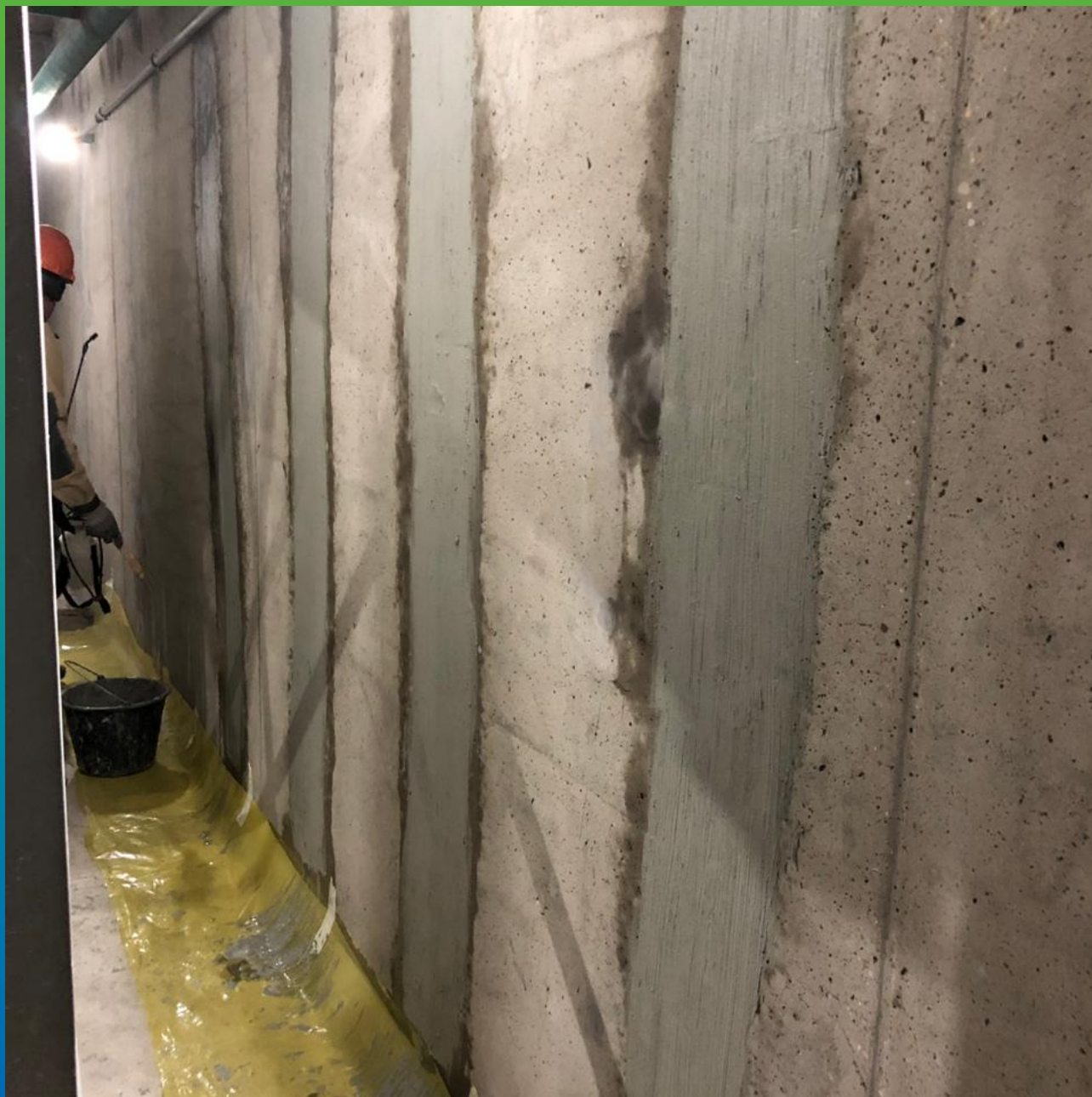
Обмазка трещин составом Стармекс Сил Флекс
