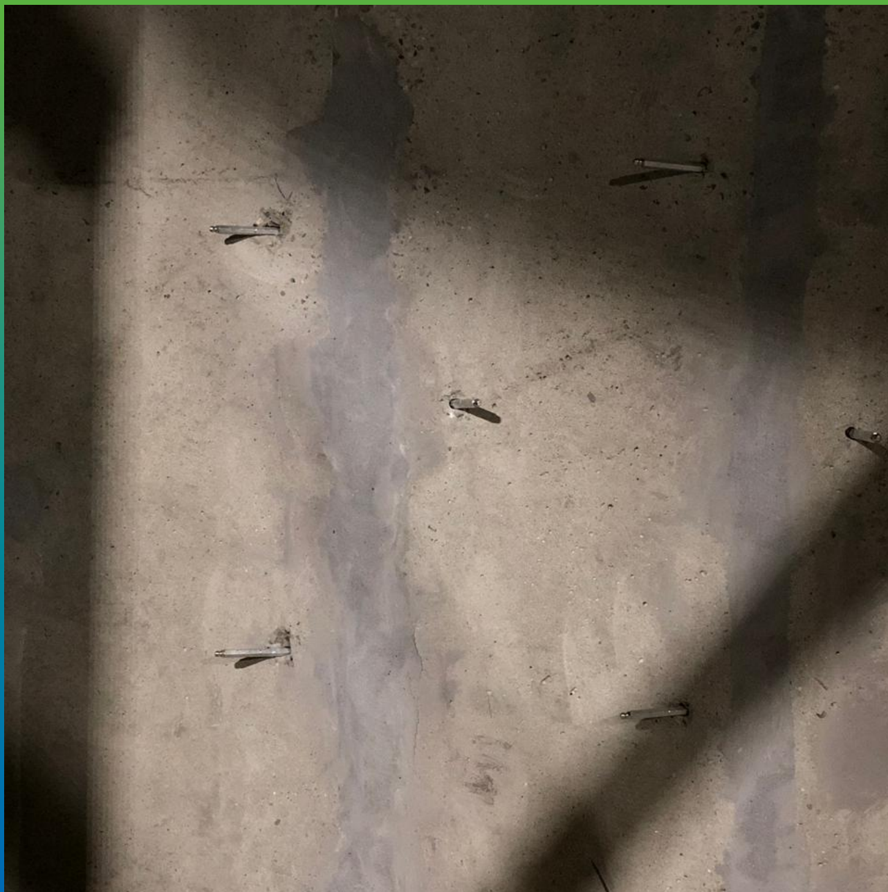
Инъектирование трещин составом Манопур 15
