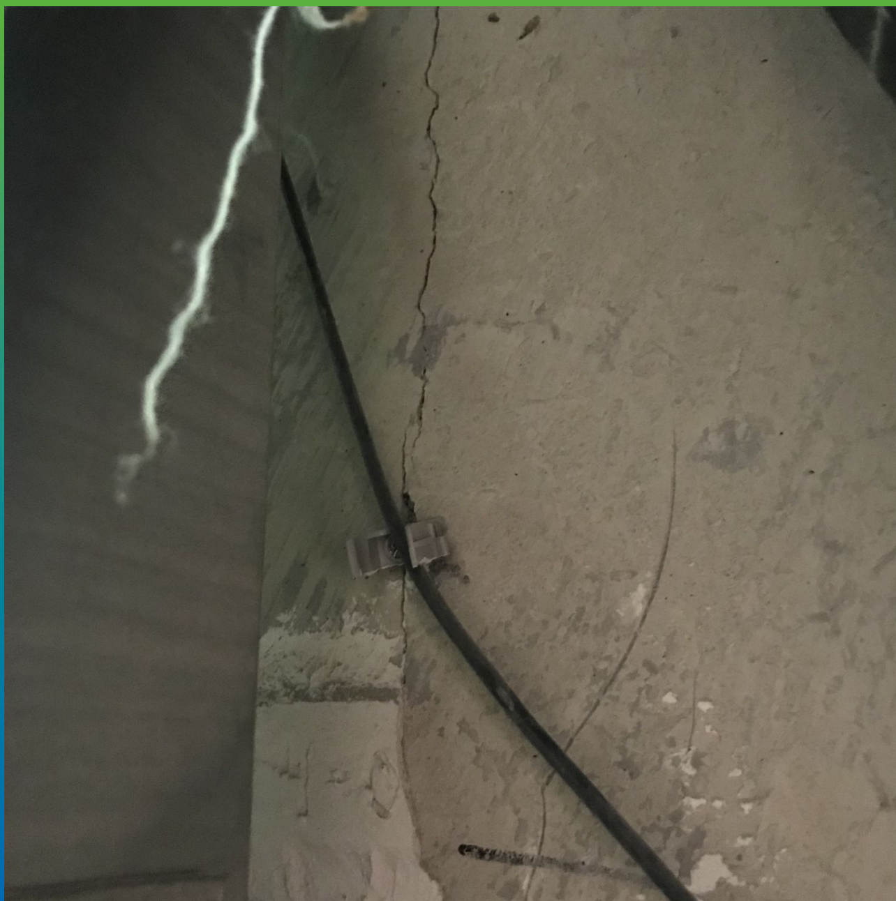
Дефекты в виде трещин, в стене и балке
