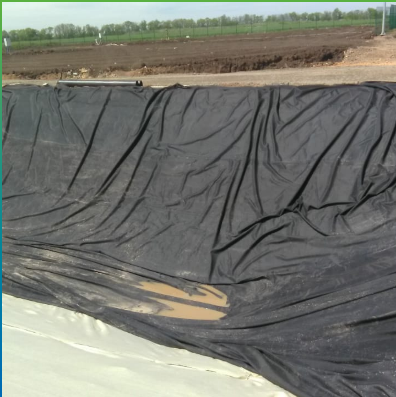
Укладка по геотекстилю цельносваренного полотна ЭПДМ
