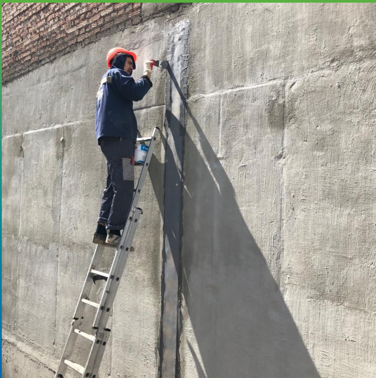
Монтаж ленты Манодил Про на клей Манопокс 331
