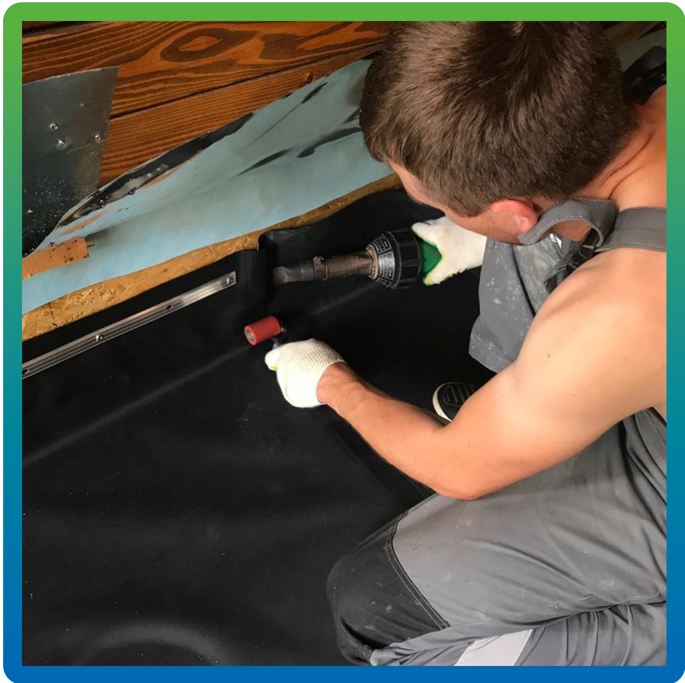
Сварка швов мембраны с помощью сварочного аппарата Leister
