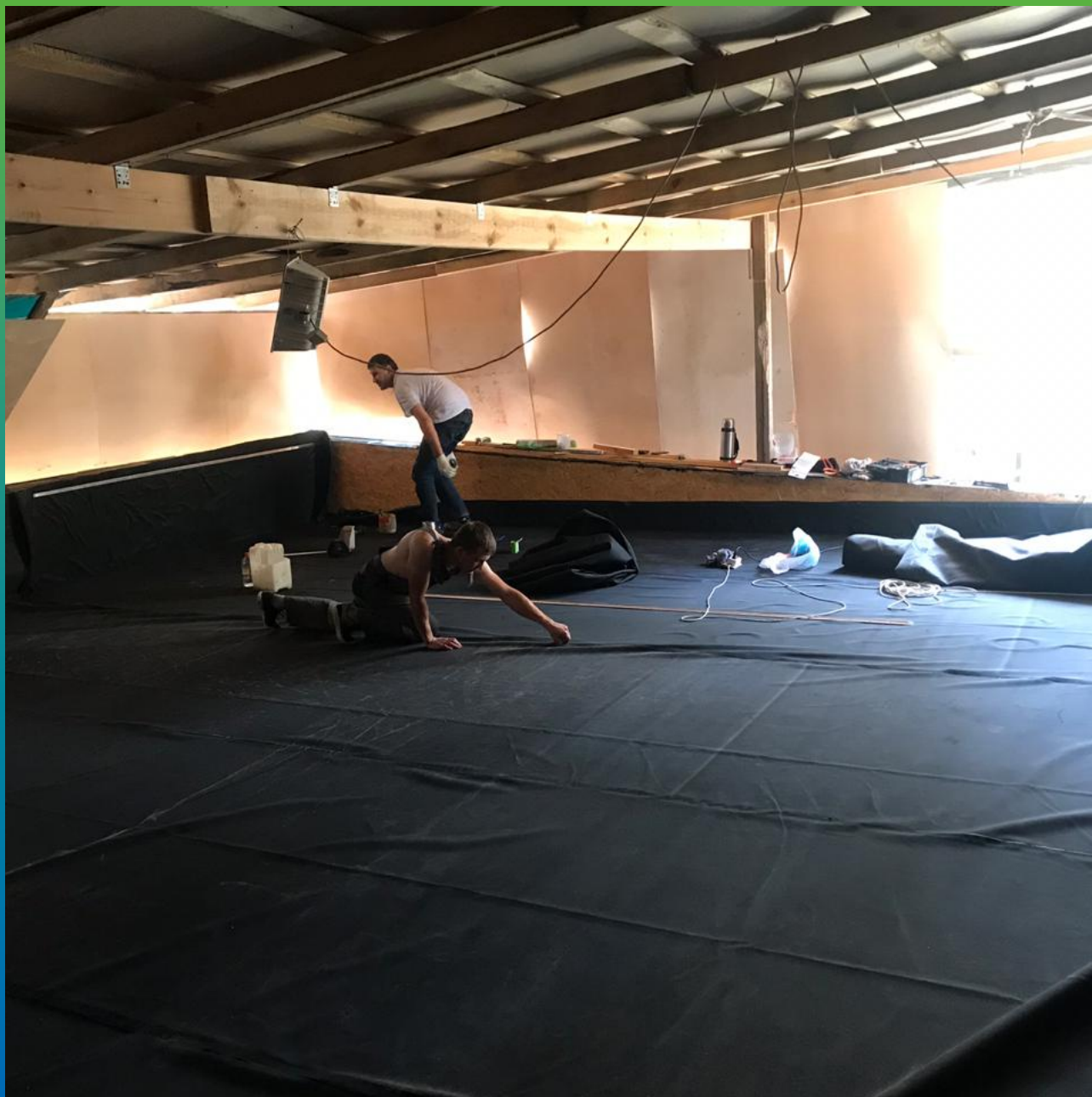
Расстилка карт мембраны и стыковка швов
