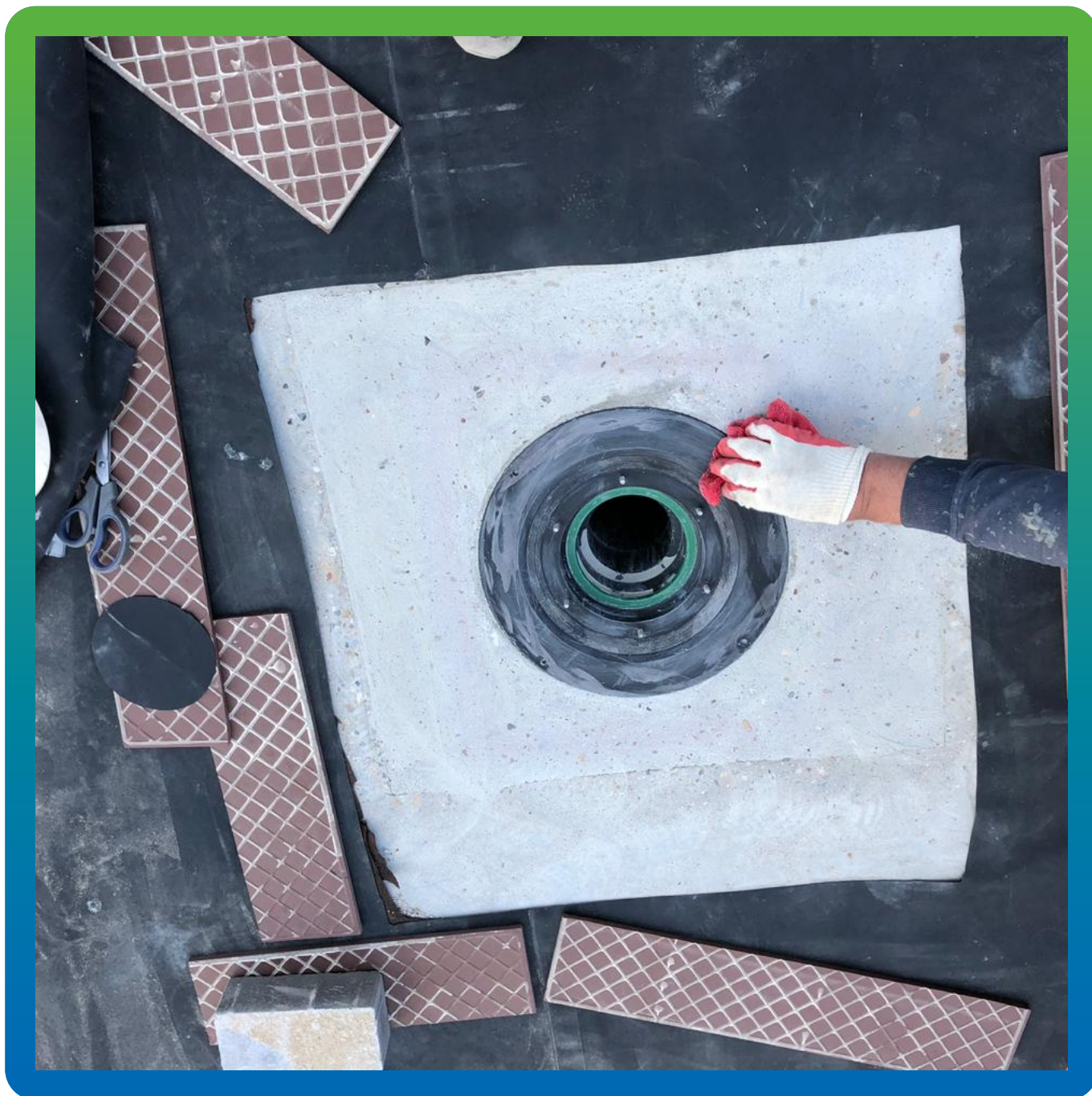
Подготовка сливной воронки к последующей гидроизоляции
