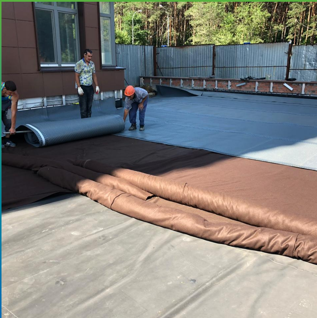
Защита уложенной мембраны геотекстилем и дренажным полотном
