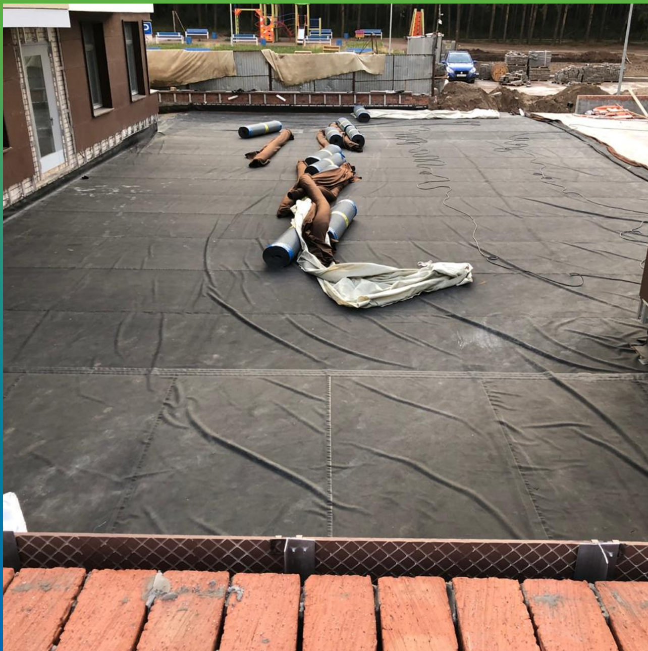
Геотекстиль и дренажное полотно для последующей защиты
