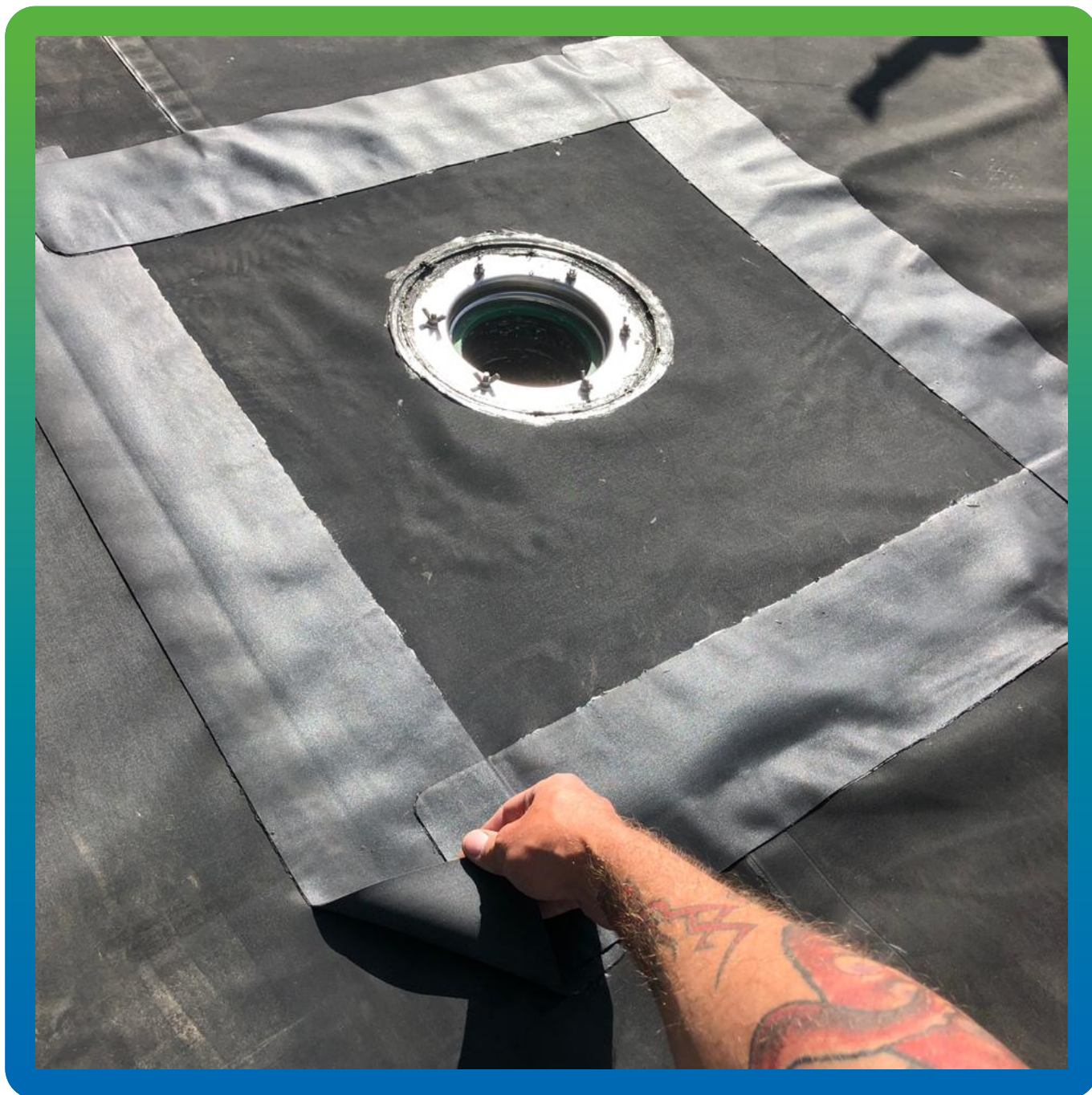
Герметизация стыков сливной воронки с картой при помощи ленты Термобонд
