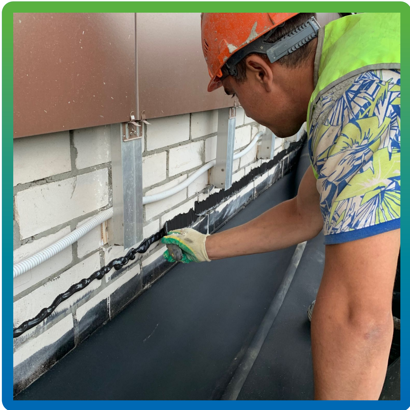
Крепление заведенных на стену кромок мембраны при помощи герметика Витрафин Бонд Ф
