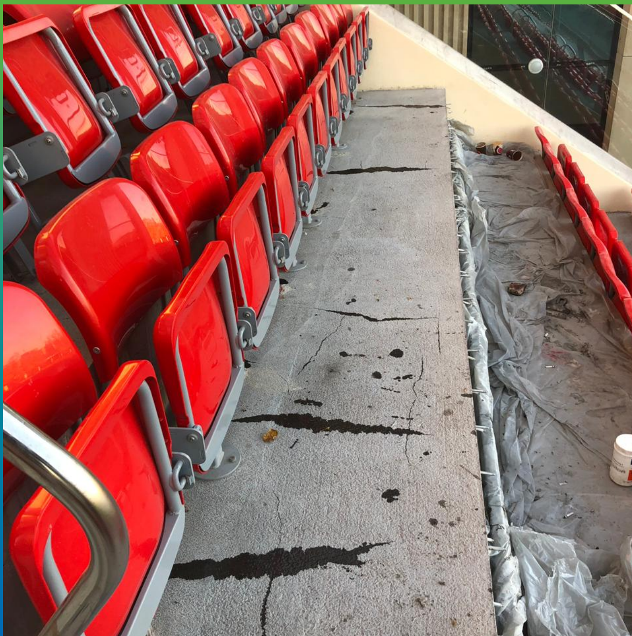
Состав Манопокс 352 выступает после нагнетания из микротрещин
