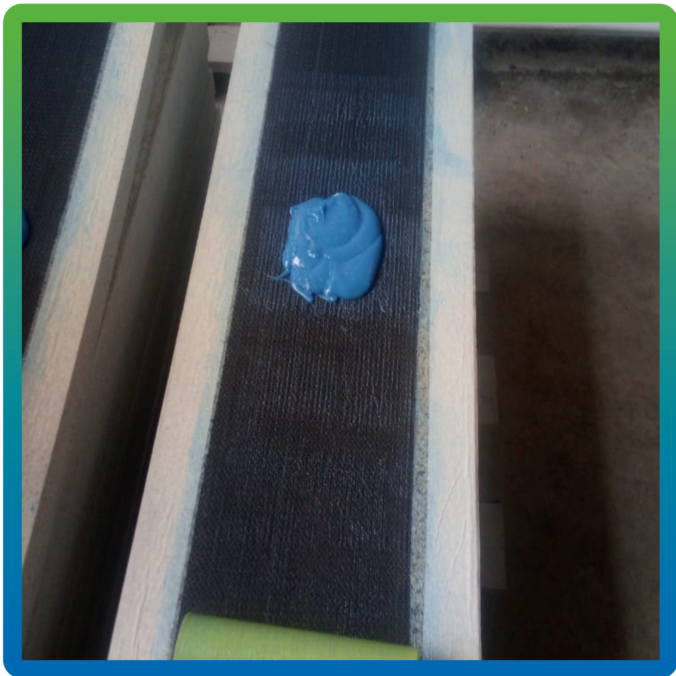
Нанесение запечатывающего слоя клея Манопокс 183.
