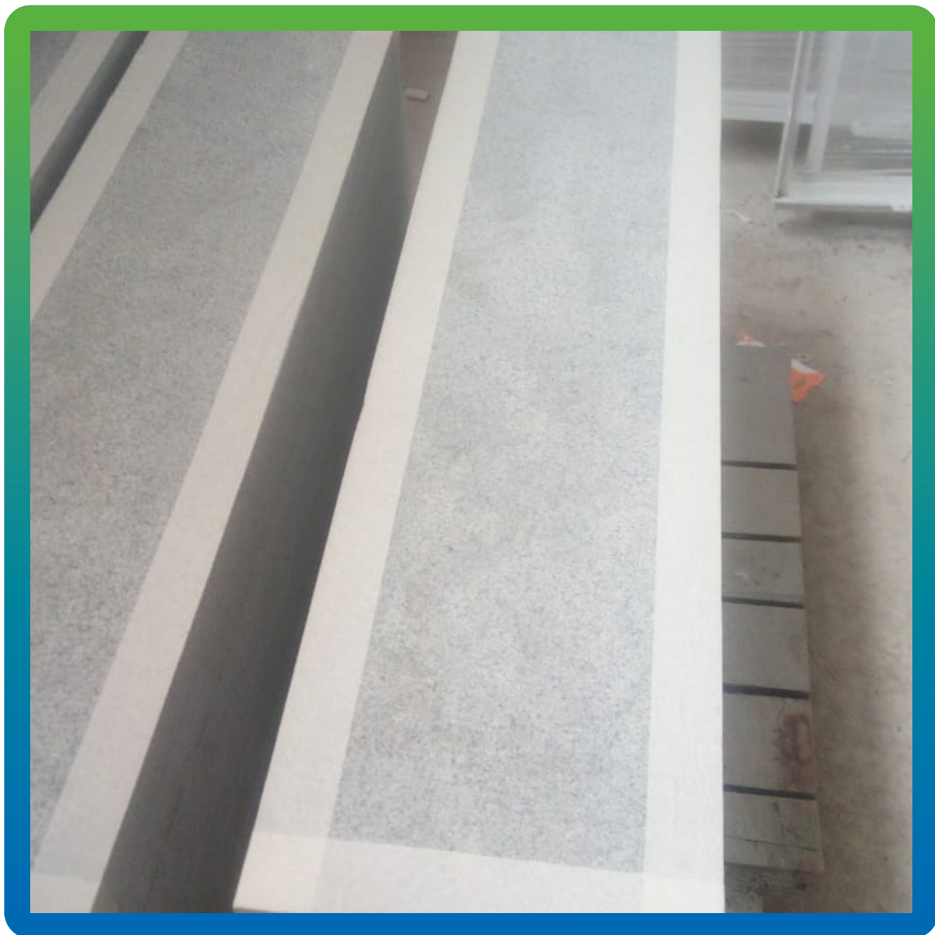
Оконтуривание поверхности под нанесение КСУ.
