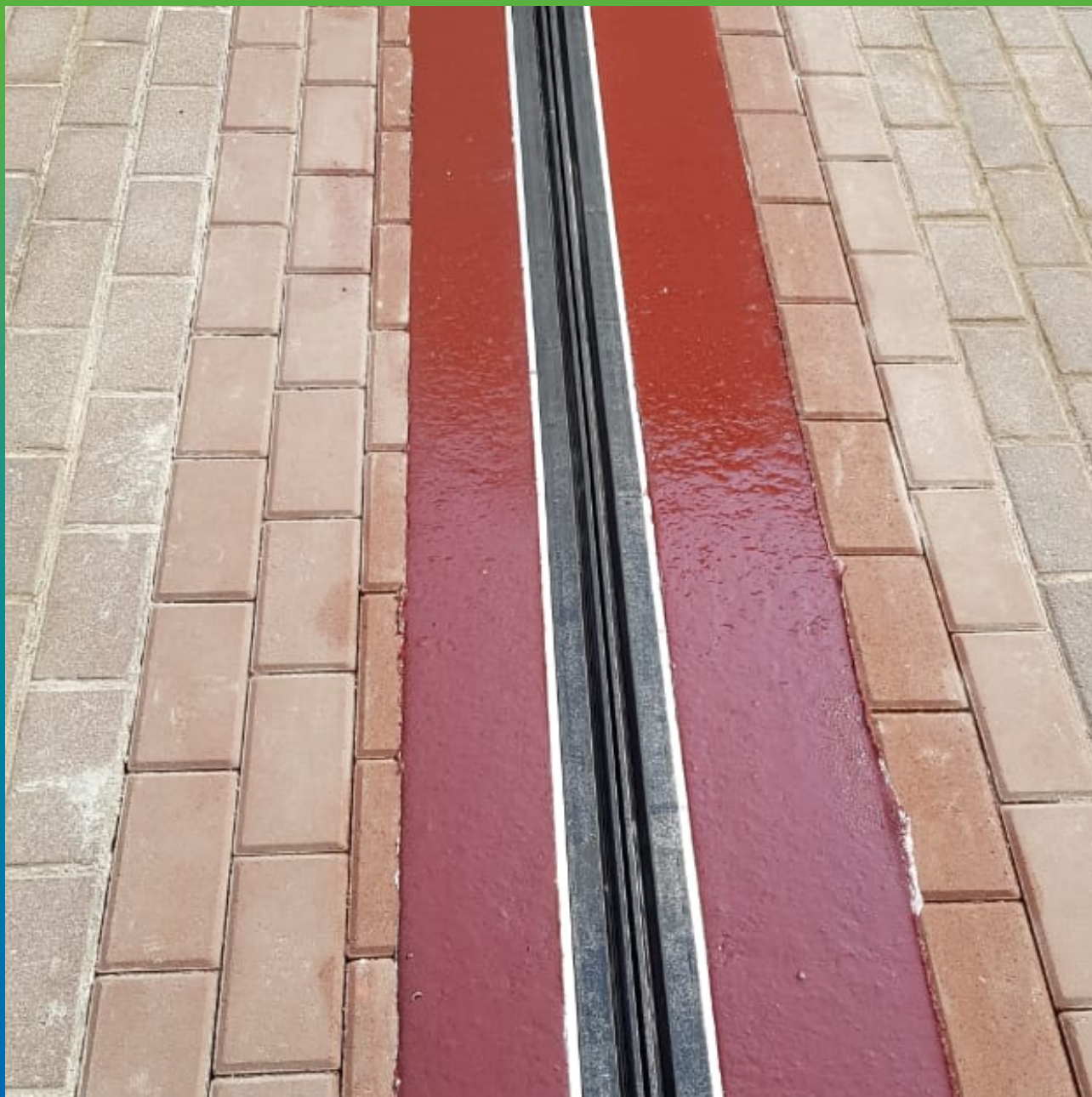
Финишный вид деформационного шва после монтажа Манопур 336
