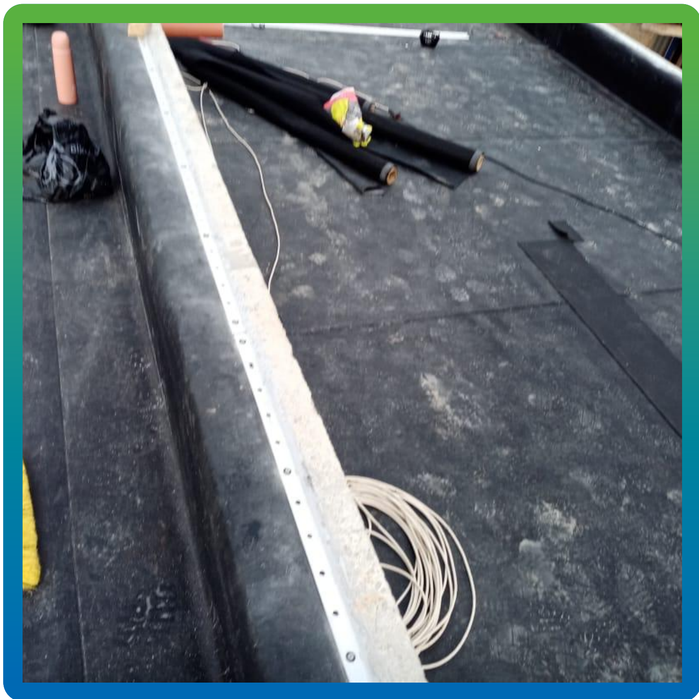
Гидроизоляция угловых элементов кровли
