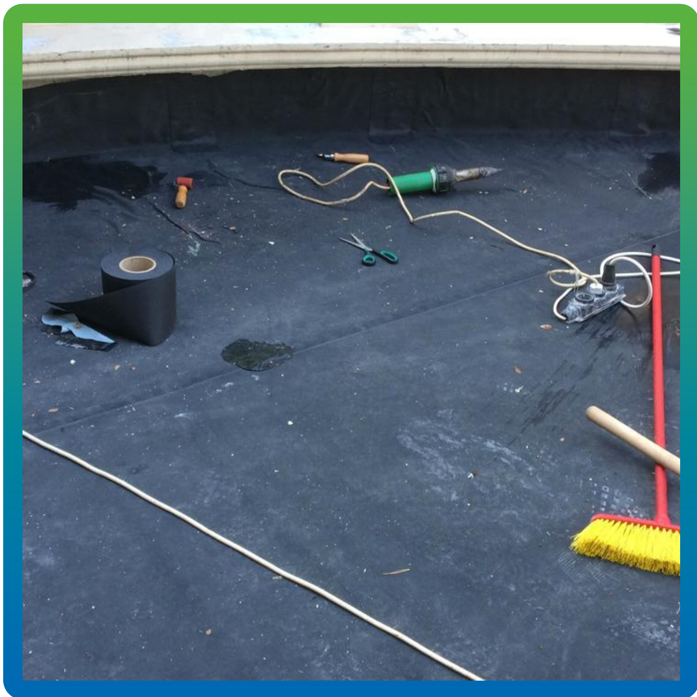
Зона примыкания - монтаж краевых реек
