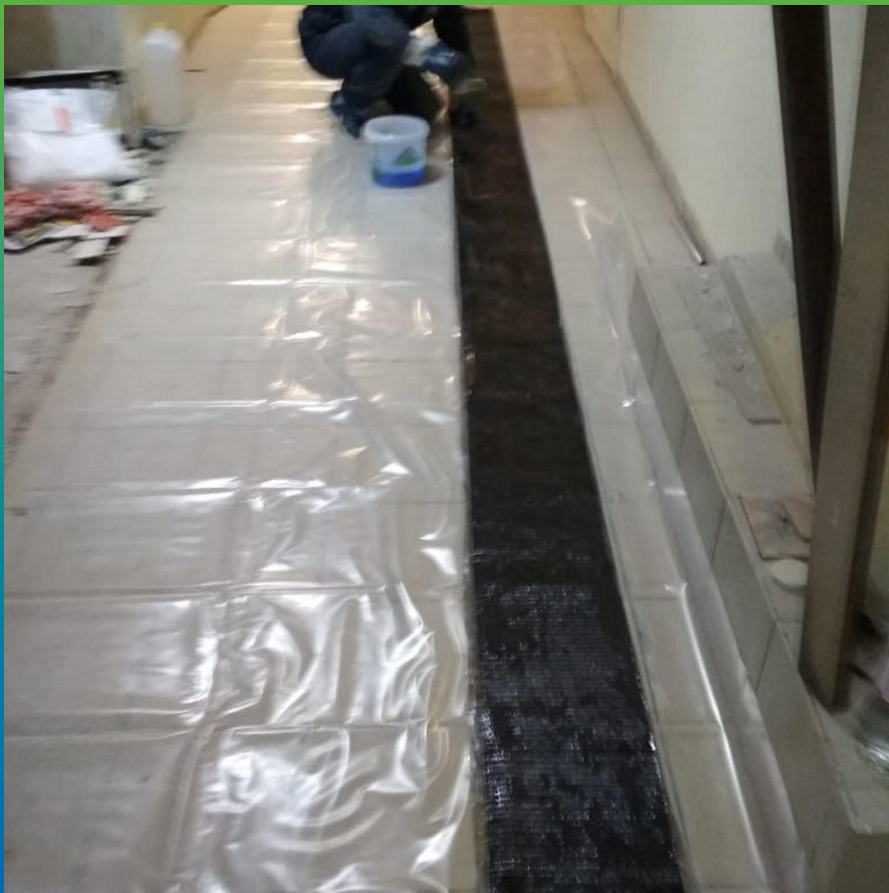
Раскрой холстов Армошел КВ 900 согласно проекта
