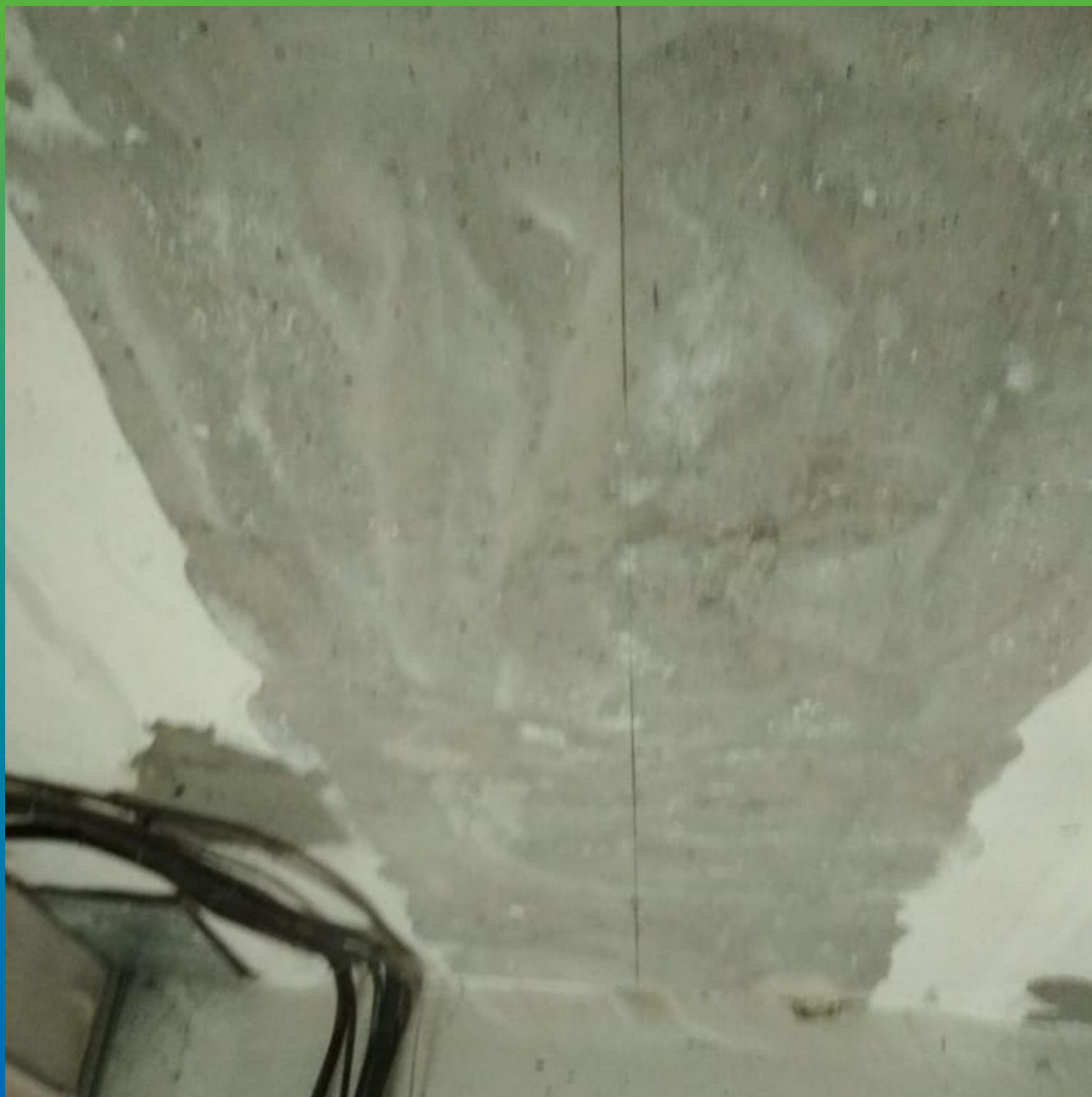
Подготовка поверхности перед монтажом "ФАП"
