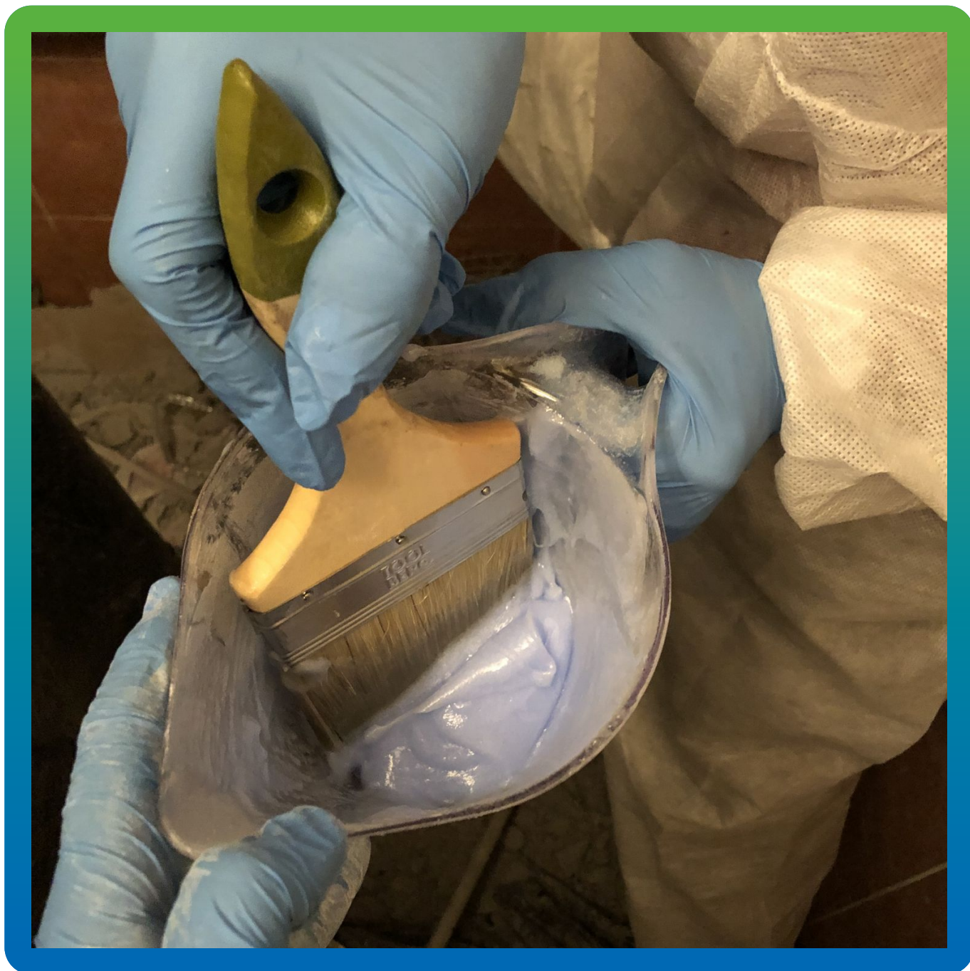
Подготовка клеевого состава Манопокс 372 + Манопокс Тикс
