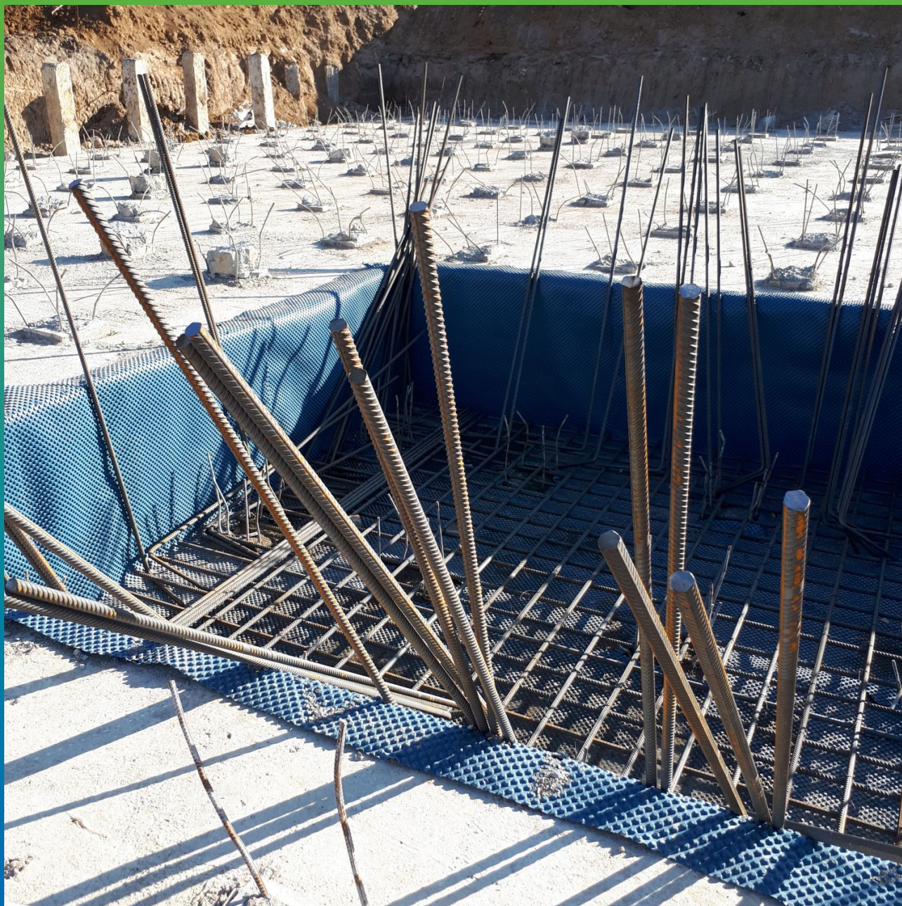
Дренажное полотно Максдрейн 8 в зоне установки башенного крана
