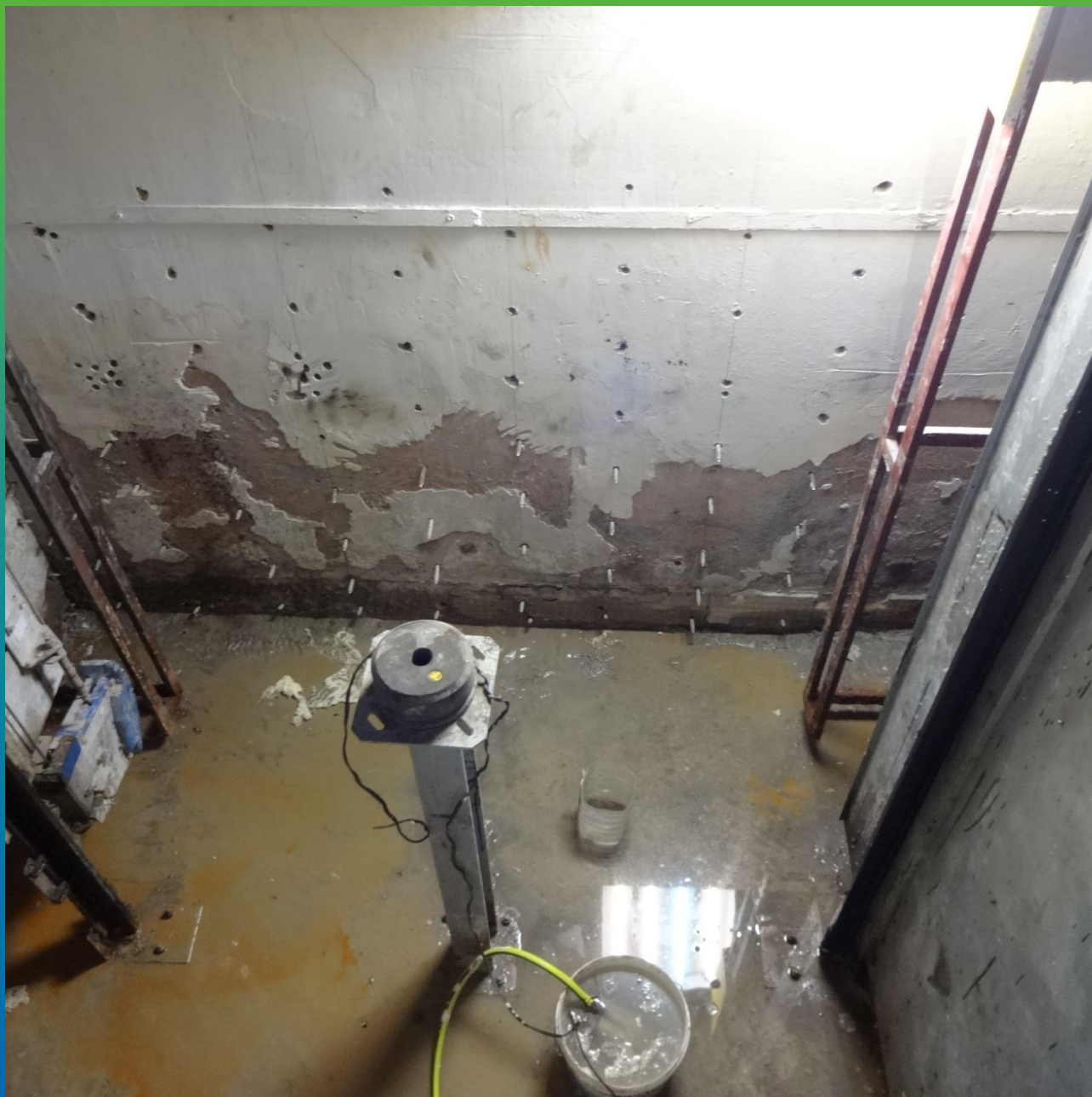
Бурение шпуров и монтаж пакеров на объекте
