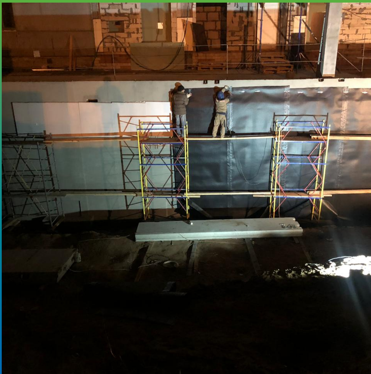
Защита гидроизоляции дренажным полотном перед обратной засыпкой.
