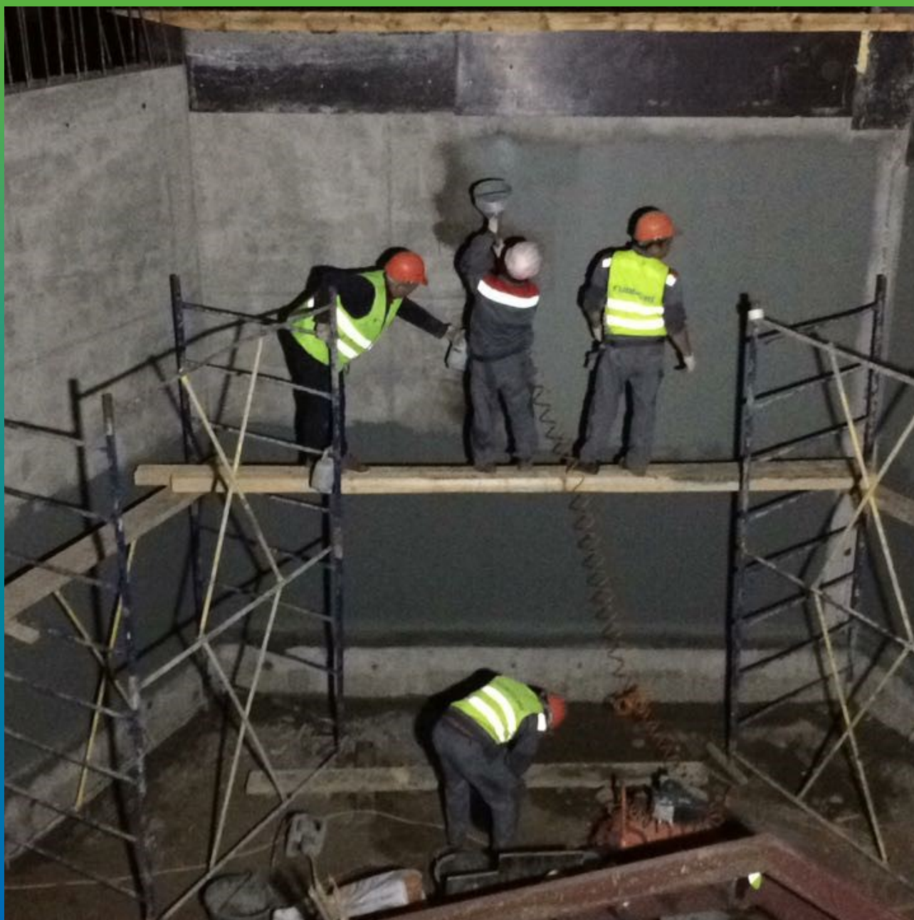
Механизированное нанесение состава Стармекс Сил Флекс.
