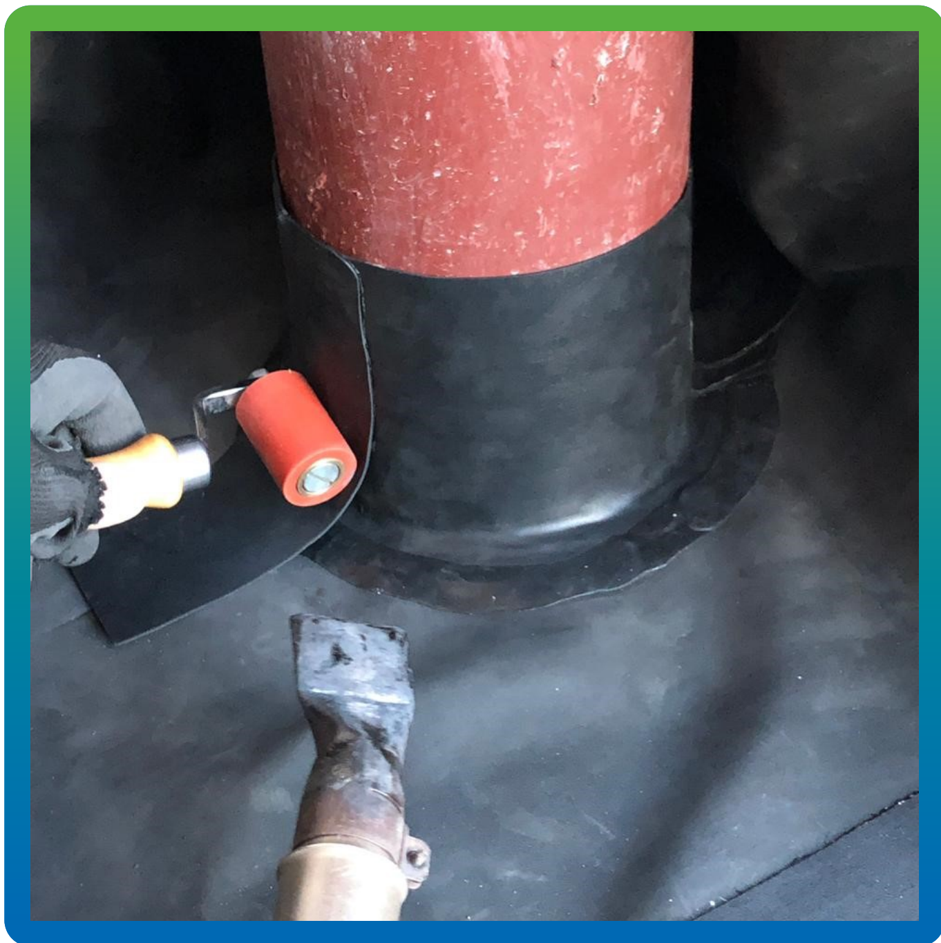
Обвод труб на гидроизолируемой поверхности
