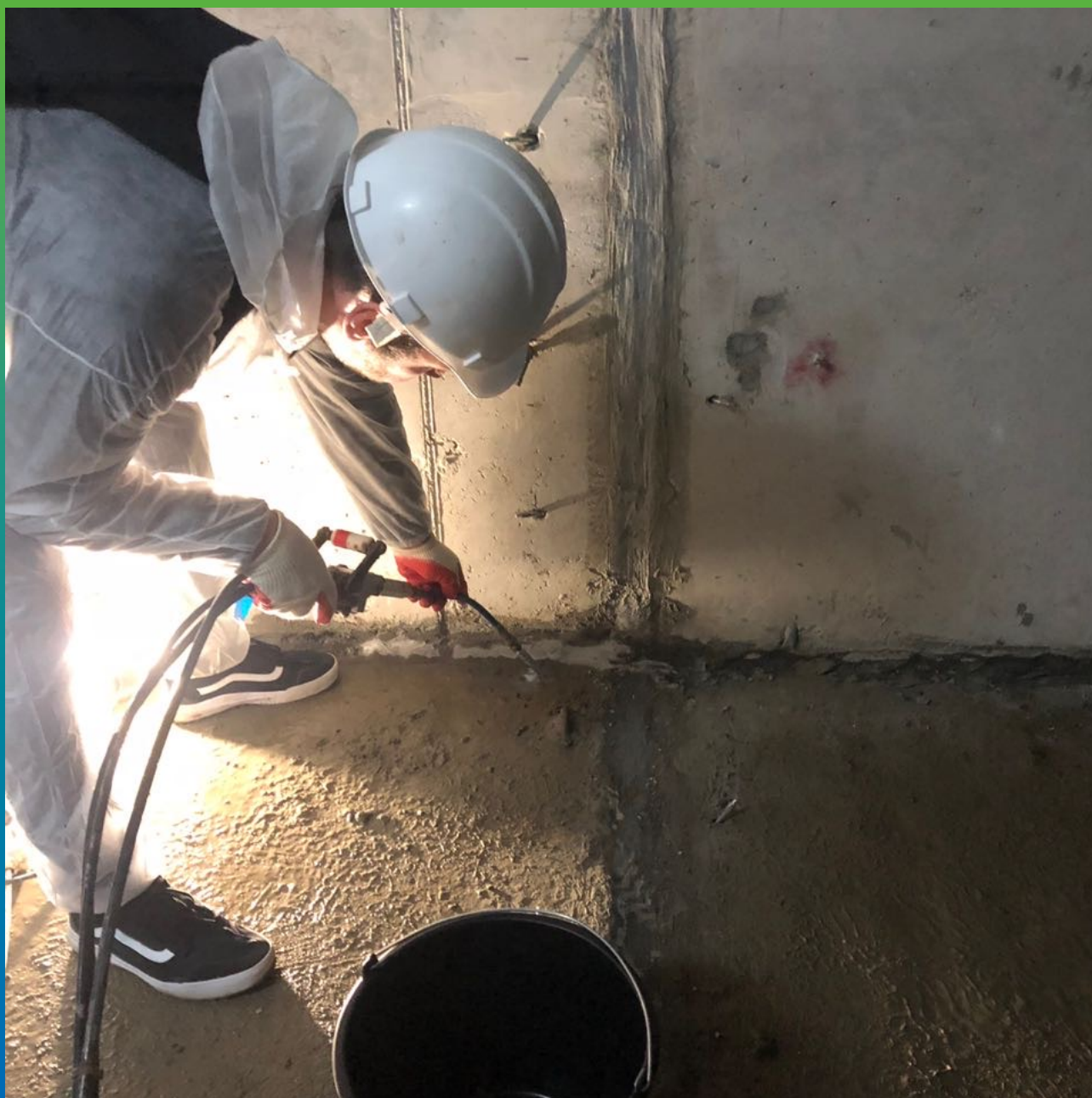
Инъектирование деформационного шва
